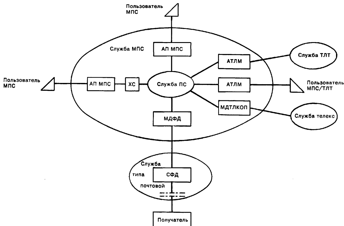
Рисунок 7 — Функциональная модель службы МПС
