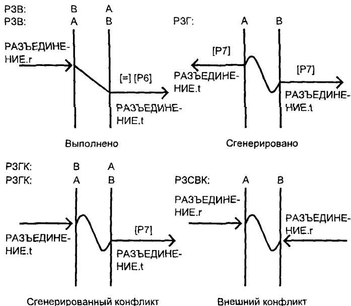
Рисунок 9 — Фаза «разъединение ССУ»
