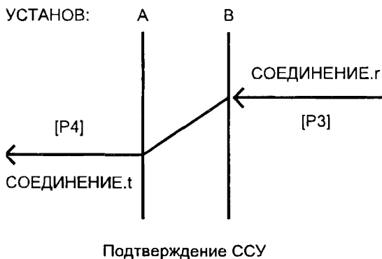
Рисунок 6 — Установление ССУ, подфаза «подтверждение ССУ»
