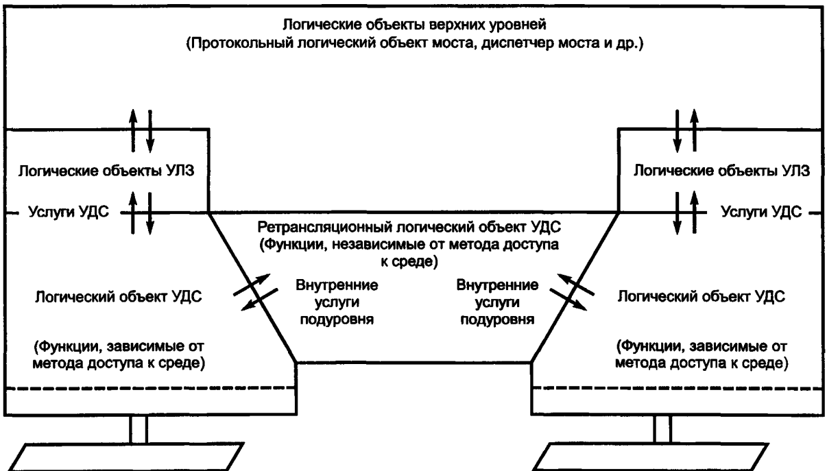
Рисунок 3.3 — Архитектура моста
