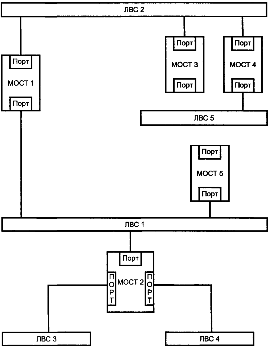
Рисунок 4.1 — Активная топология
