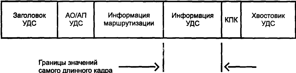
Рисунок С.6 — Границы значений самого длинного кадра
