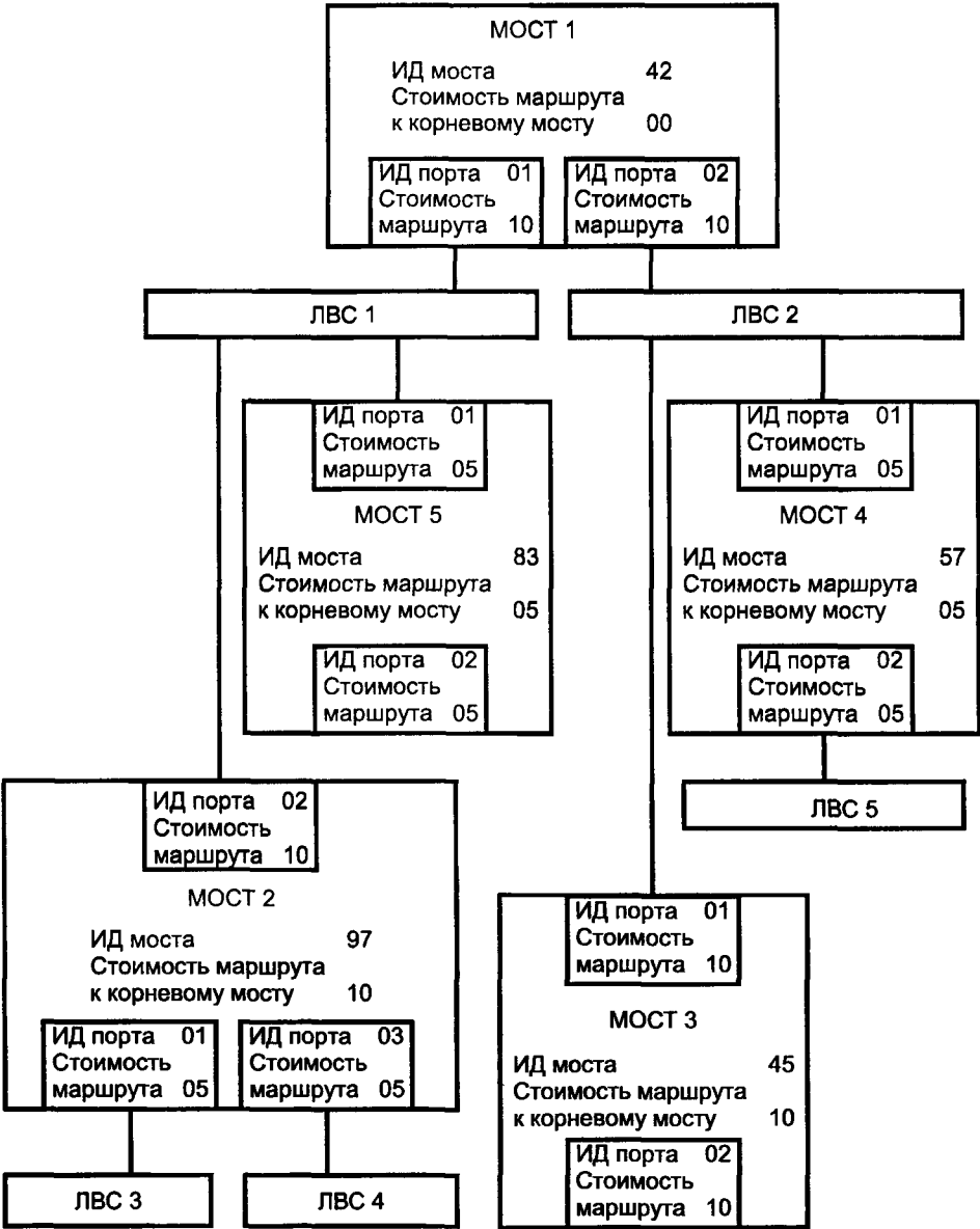
Рисунок 4.2 — Связующее дерево
