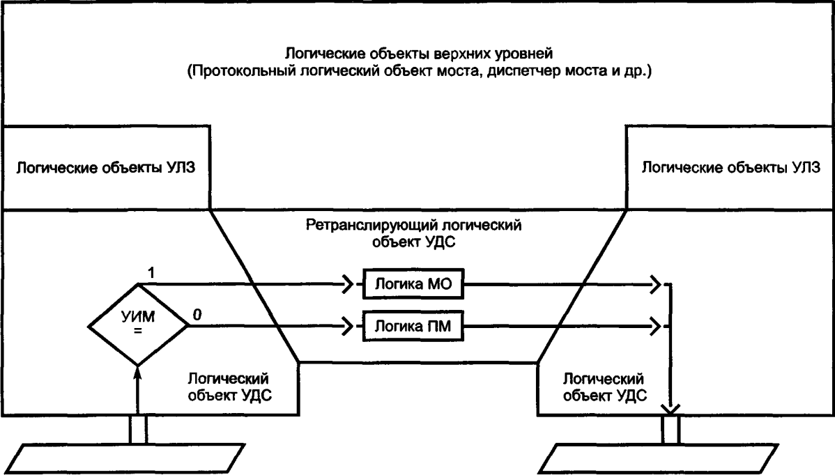
Рисунок С.1 — Логика операций моста ПМСО
