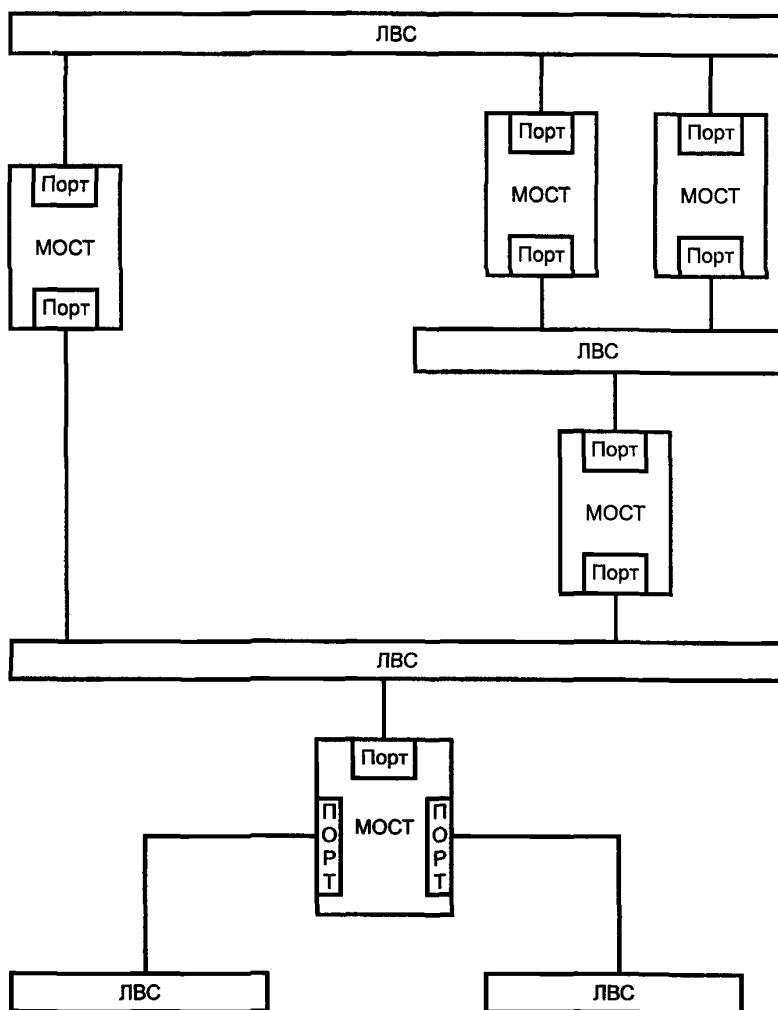
Рисунок 3.1 — Мостовая локальная вычислительная сеть
