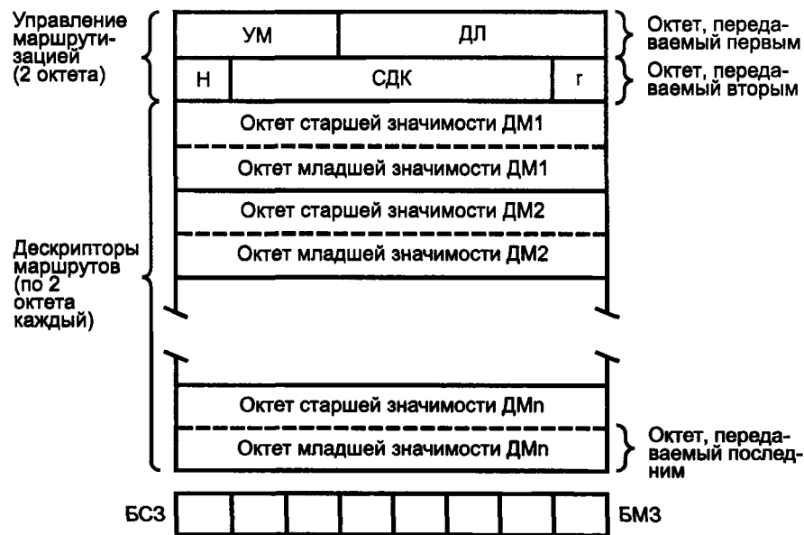
Рисунок С.3 — Поле информации маршрутизации
