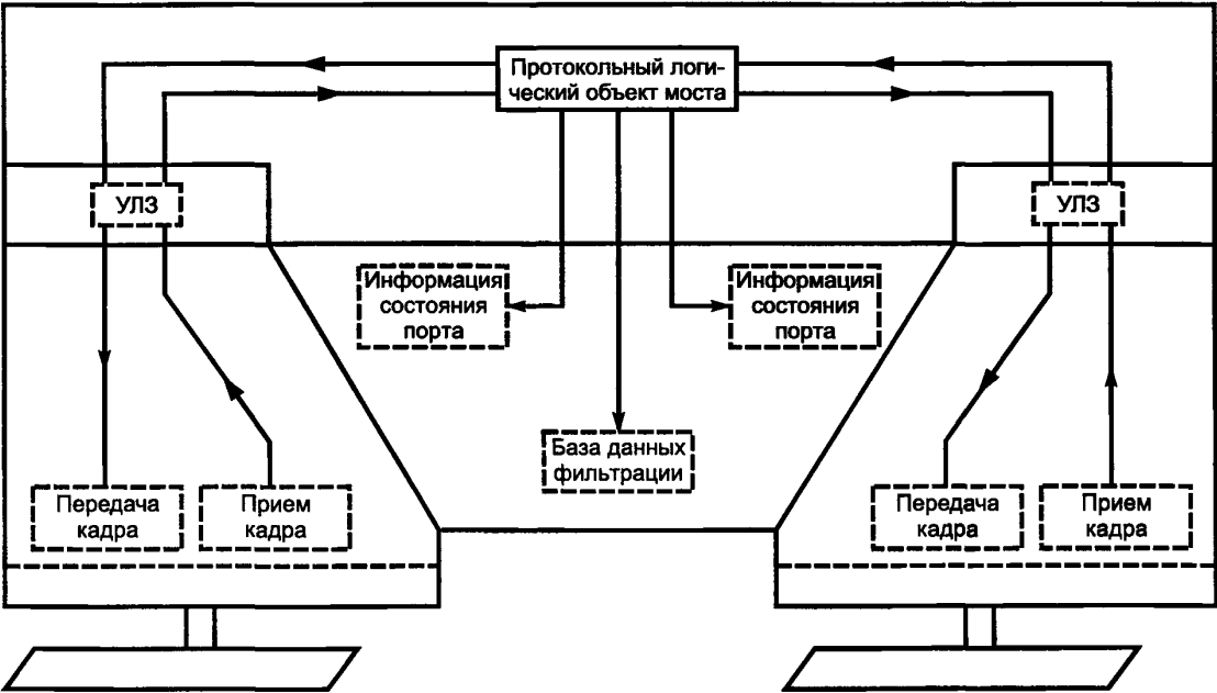
Рисунок 3.6 — Операции межмостового протокола
