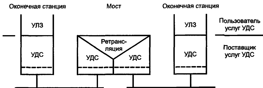
Рисунок 2.1 — Внутренняя организация подуровня УДС
