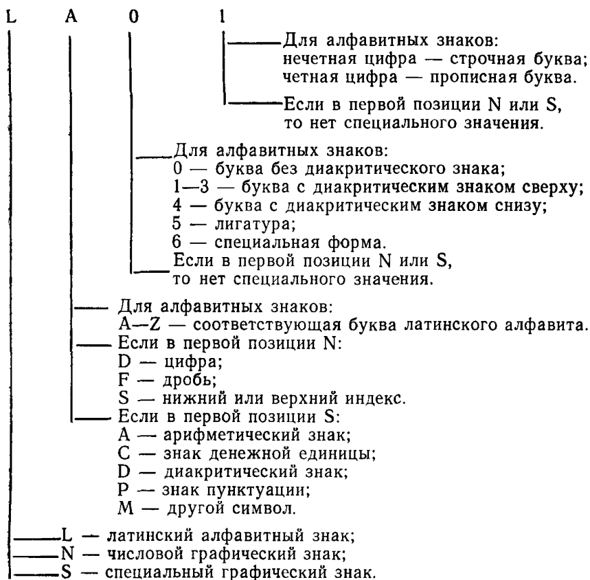
Рисунок В.1 — Метод определения коротких идентификаторов
