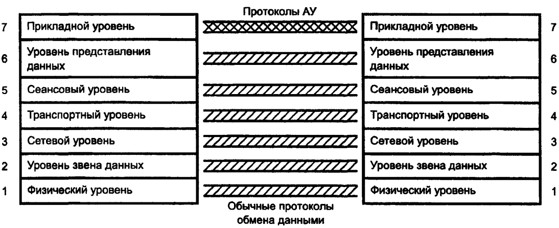
Рисунок А.1 — Обмен информацией АУ систем
