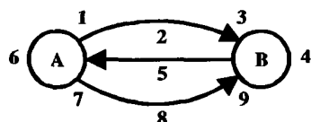
Рисунок 9 — Трехнаправленная аутентификация
