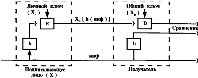
Рисунок 6 — Цифровые подписи
