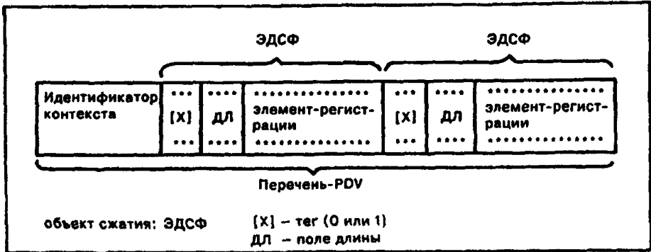
Рисунок 5 — Метод сжатия INTAP-СП1
