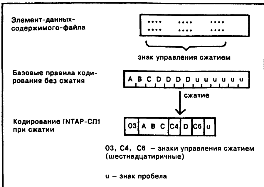
Рисунок 7 — Пример кодирования при использовании INTAP-СП1
