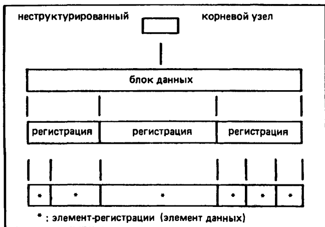
Рисунок 1 — Структура типа документа по INTAP—1
