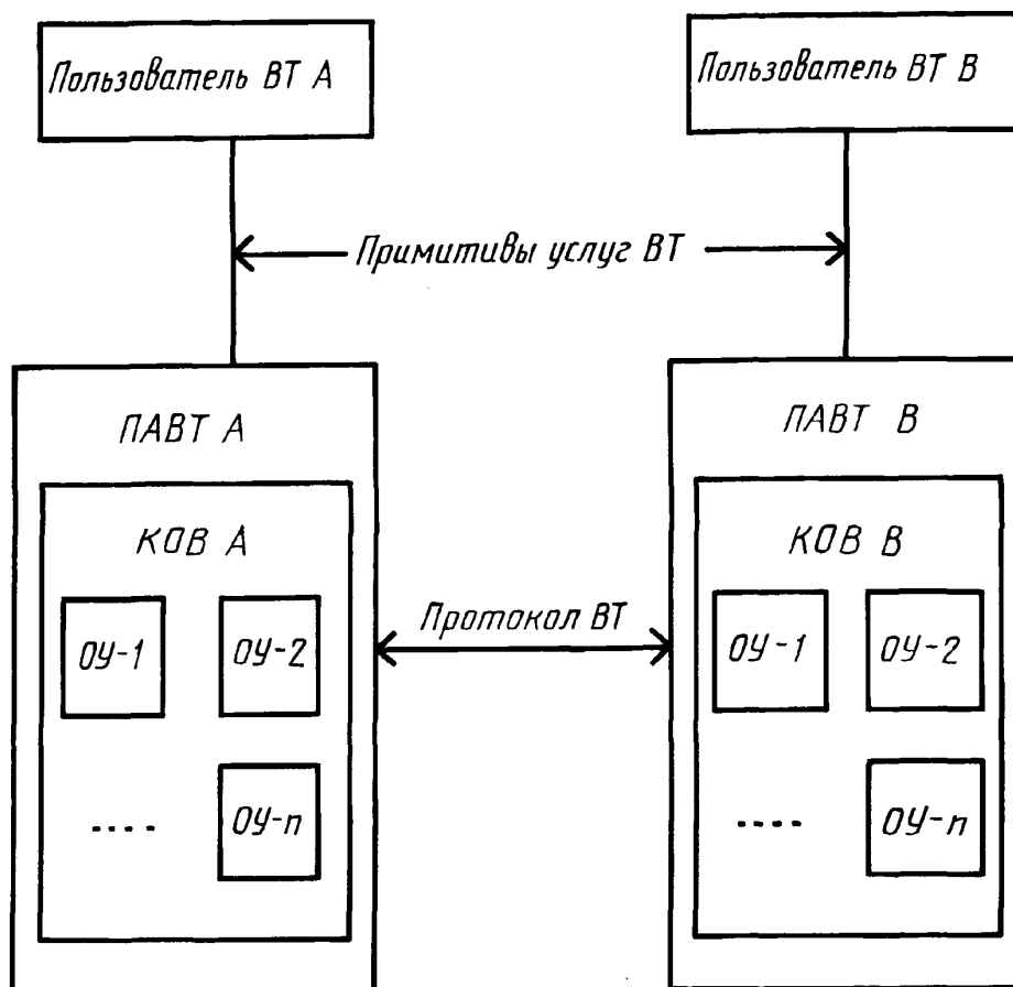
Рисунок 2 — Объекты управления в модели протокола ВТ
