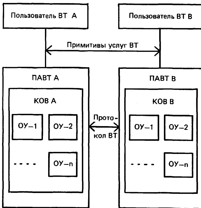
Рисунок 2 — Объекты управления в модели протокола ВТ
