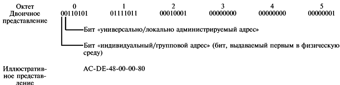
Рисунок 1 — Представление адресов УДС ЛВС
