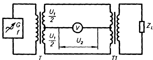
T1 — испытуемый трансформатор
