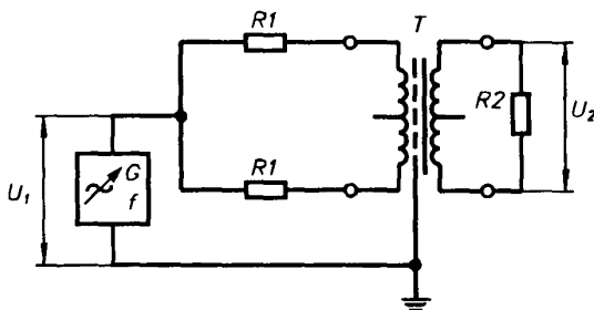
T — испытуемый трансформатор
