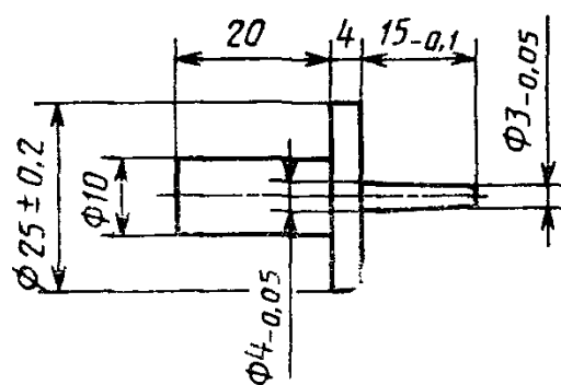
Рисунок 2 — Испытательный шуп
