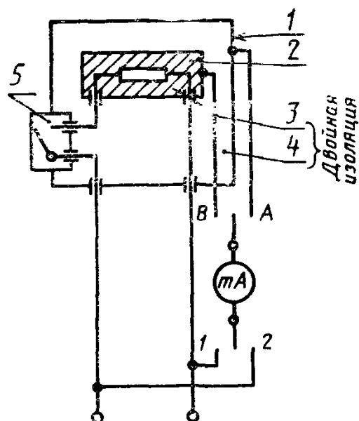
Рисунок 2 — Испытательный шуп
