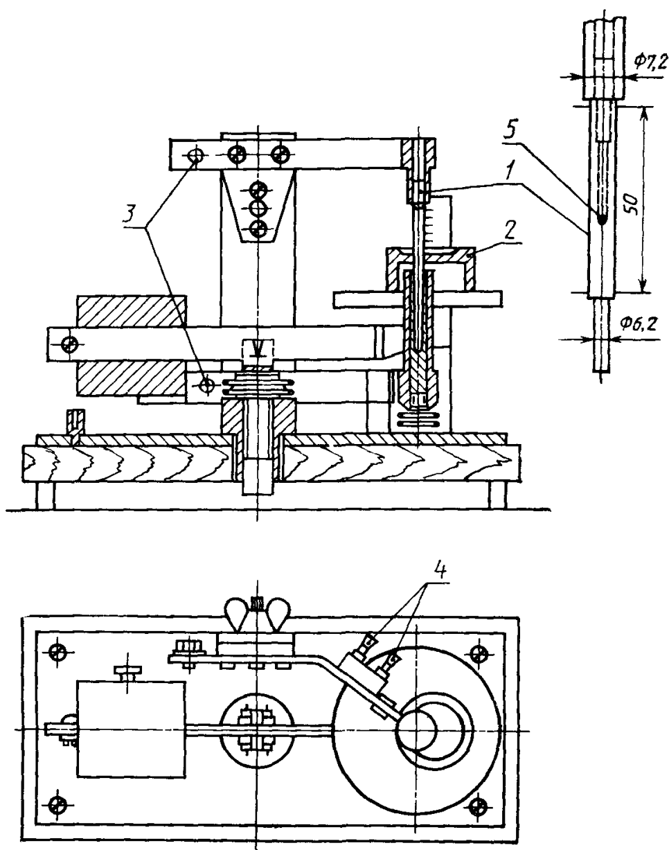
1—конический сердечник; 2—испытуемый образец; 3—зажимы для подвода тока нагрева; 4—зажимы для термопары; 5—термопара
