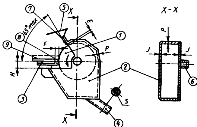
I — шлифовальный круг, 2 — защитный кожух круга, 3 — рабочий упор, 4 — мунштук для удаления пыли, 5 — прозрачный экран, 6 — ограждение оси, 7 — искрогаситель, 8 — рабочая зона круга, 9 — обрабатываемое изделие, P — толщина периферической части кожуха, J — толщина боковых стенок кожуха, S — внутреннее сечение мунштука, D — максимальный наружный диаметр круга, E — зазор между искрогасителем и кругом, F — зазор между рабочим упором и кругом
