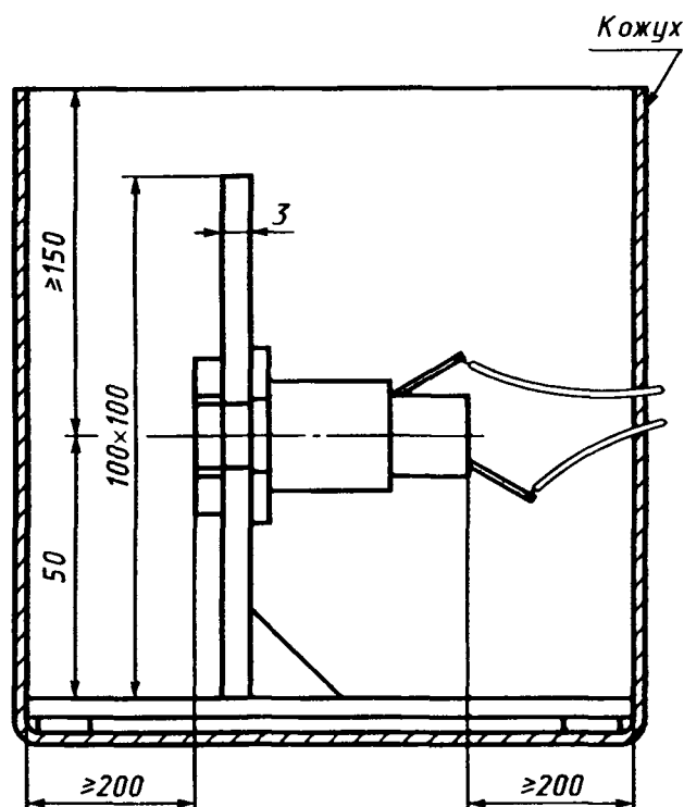
Рисунок 11 — Испытательное устройство
