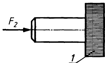
1 — поверхность компонента; F_2 — усилие сжатия
