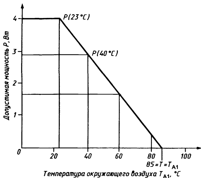
P(23^\circ\text{C}) — номинальная допустимая мощность Рисунок 12 — Пример снижения мощности
