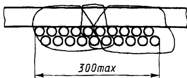
Рисунок 3г — Кабели небольшого диаметра, закрепленные на передней стороне стандартной лестницы (сформированные в пучки, кодовое обозначение A (F))
