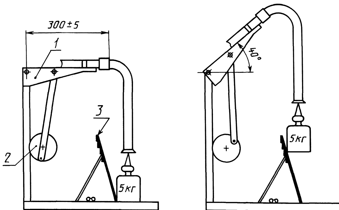
1 — качающийся рычаг; 2 — кривошипный механизм; 3 — наклонная плоскость
