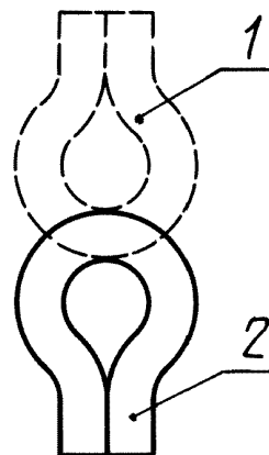
1 — промежуточное положение; 2 — положение шланга в начале и конце каждого изгибания
