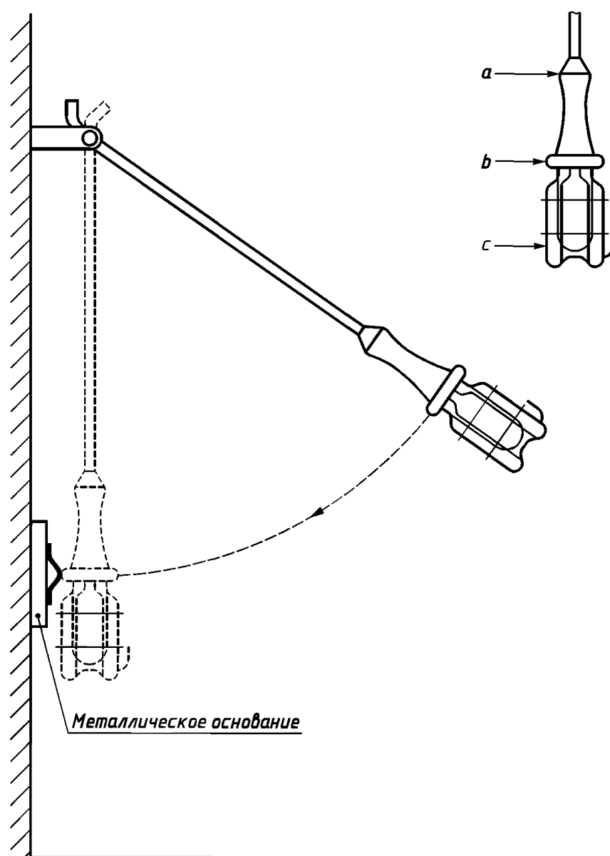
Рисунок 1 — Устройство для испытания светильников на удар
