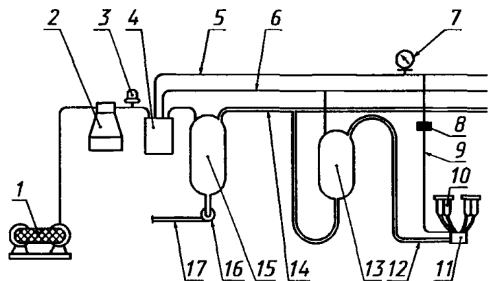
Рисунок АА 2 — Доильная установка с подачей молока непосредственно в бидон
