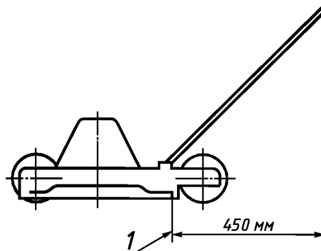
1 — траектория лезвия
