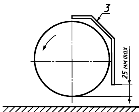
Рисунок 107 — Укрытие сторон барабанов
