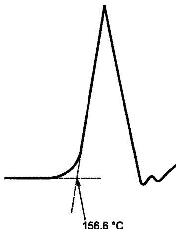
Рисунок В.1 — Типичная эндотерма плавления индия
