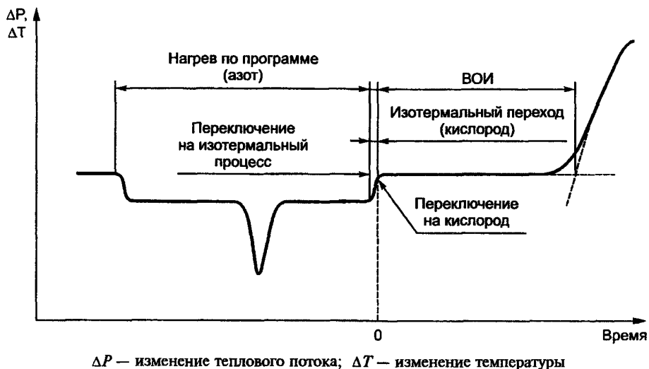
Рисунок В.2 — Определение ВОИ по термограмме
