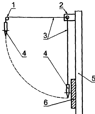
1 — исходная точка; 2 — точка крепления; 3 — шнур; 4 — электрический шуп; 5 — стена; 6 — доска из твердых пород дерева
