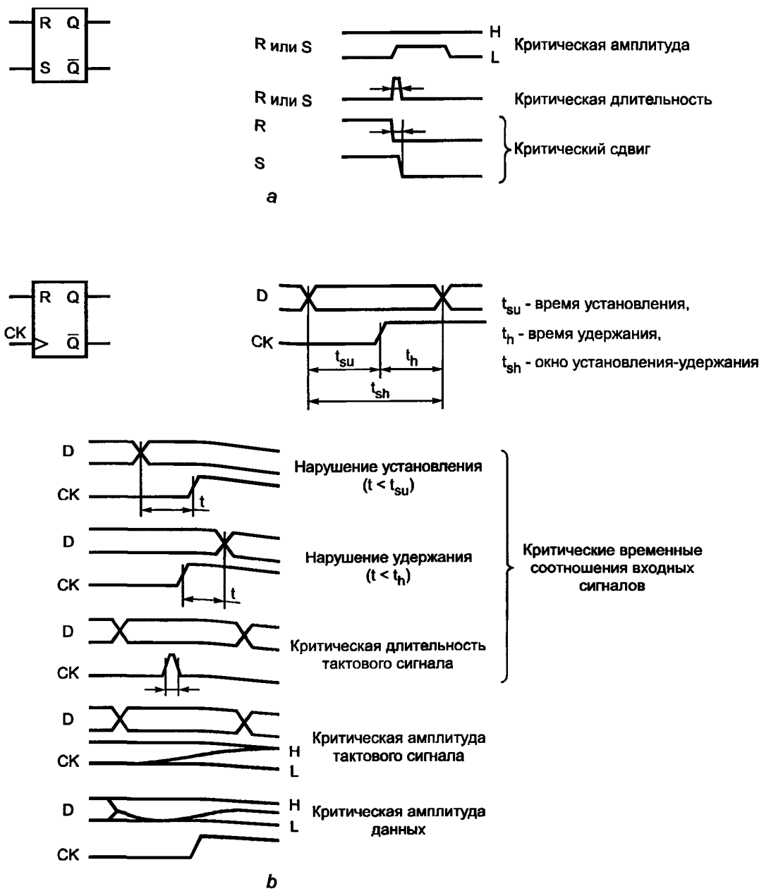
а) RS-триггер; б) D-триггер.
