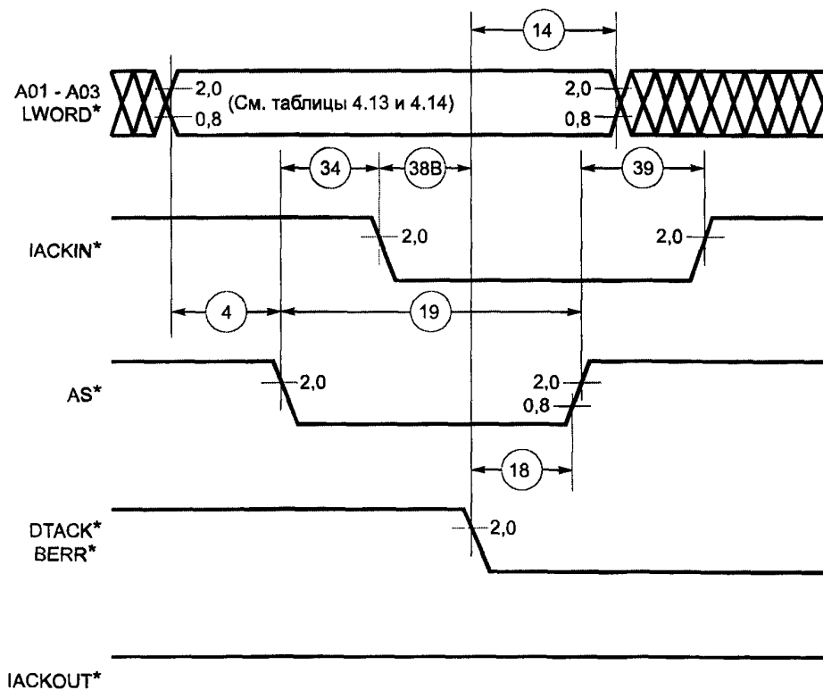
Значения напряжения пороговых уровней указаны в вольтах
