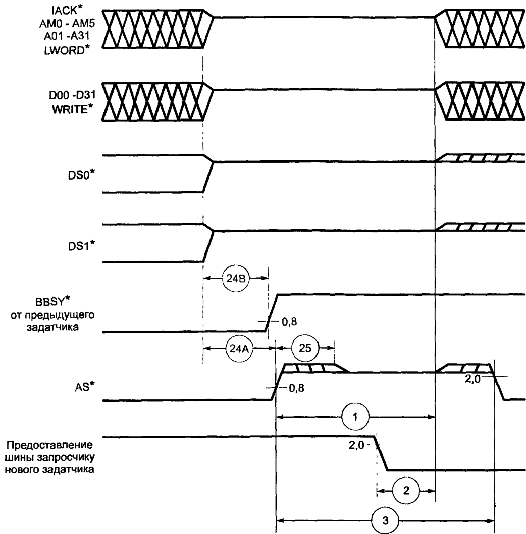
Рисунок 2.26 содержит временные диаграммы во время передачи управления шиной пересылки данных.
