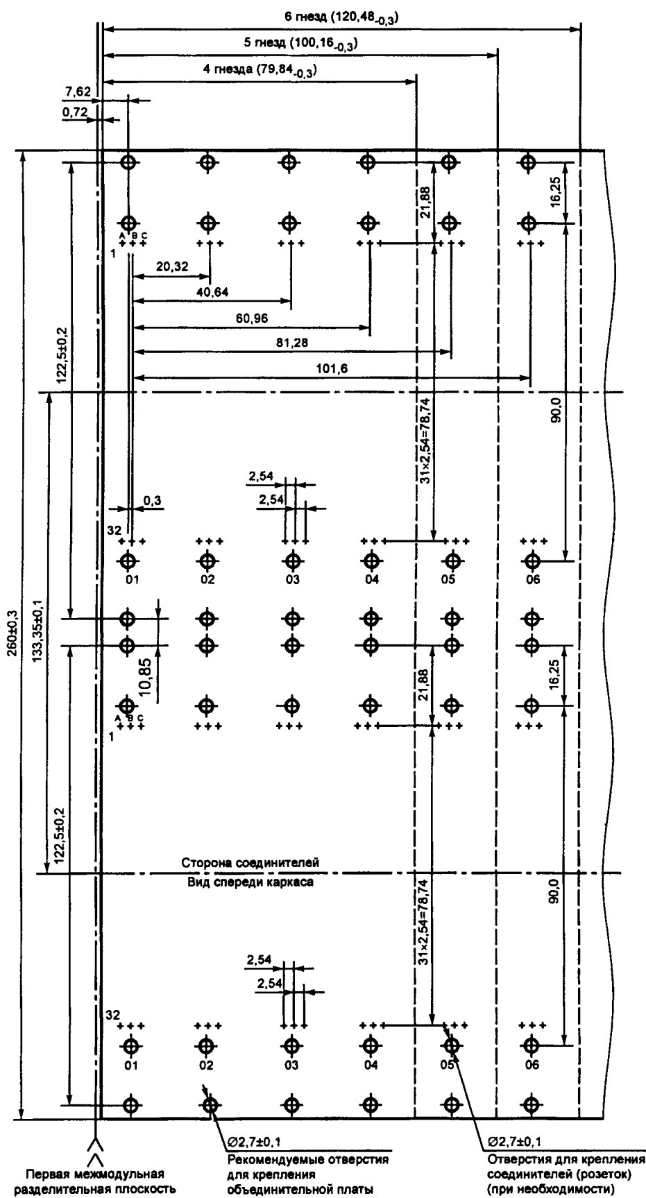
Рисунок 7.16 — Детальные размеры комбинированной объединительной платы J1/J2
