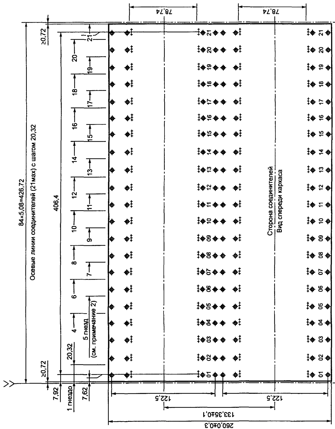
Примечания 1 Газрешение 7.24. Высота объединительной платы J1/J2 МОЖЕТ составлять (262,05 \pm 0,3) мм. 2 Ширина объединительной платы зависит от количества гнезд. Рисунок 7.15 — Габаритные и присоединительные размеры комбинированной объединительной платы J1/J2
