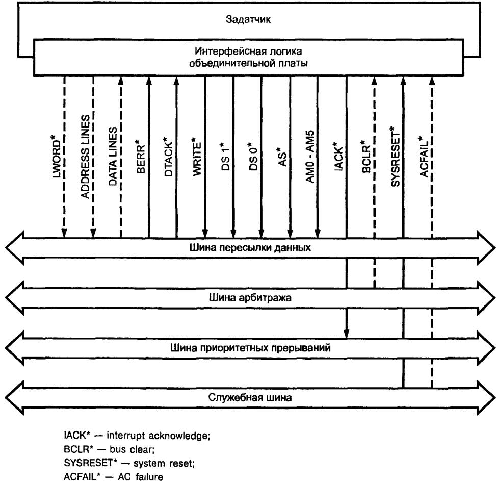
Рисунок 2.2 — Схема взаимодействия задатчика с магистралью
