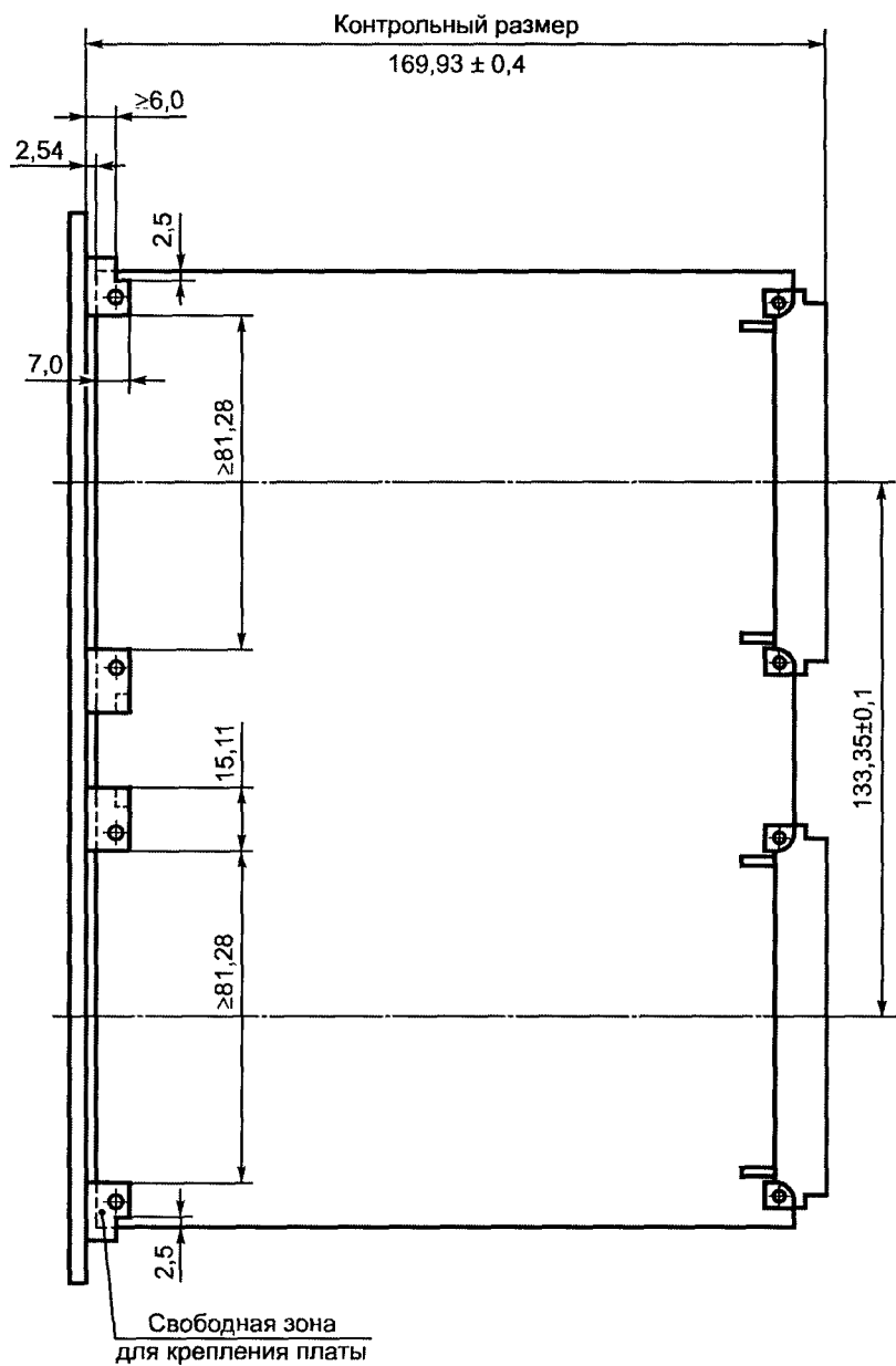
Рисунок 7.10 — Крепежные угольники передней панели и размеры модуля двойной высоты
