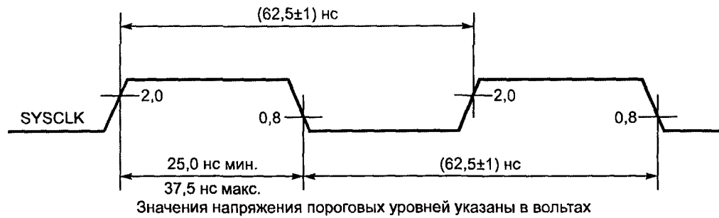
Рисунок 5.2 — Временная диаграмма работы формирователя системного тактового сигнала
