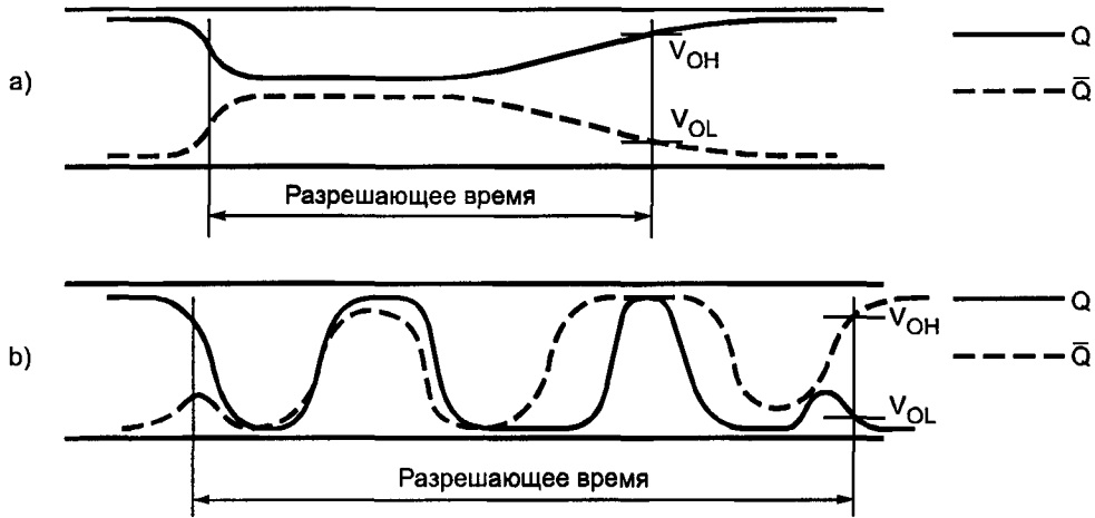
а) — аналоговая метастабильность; б) — колебательная метастабильность.
