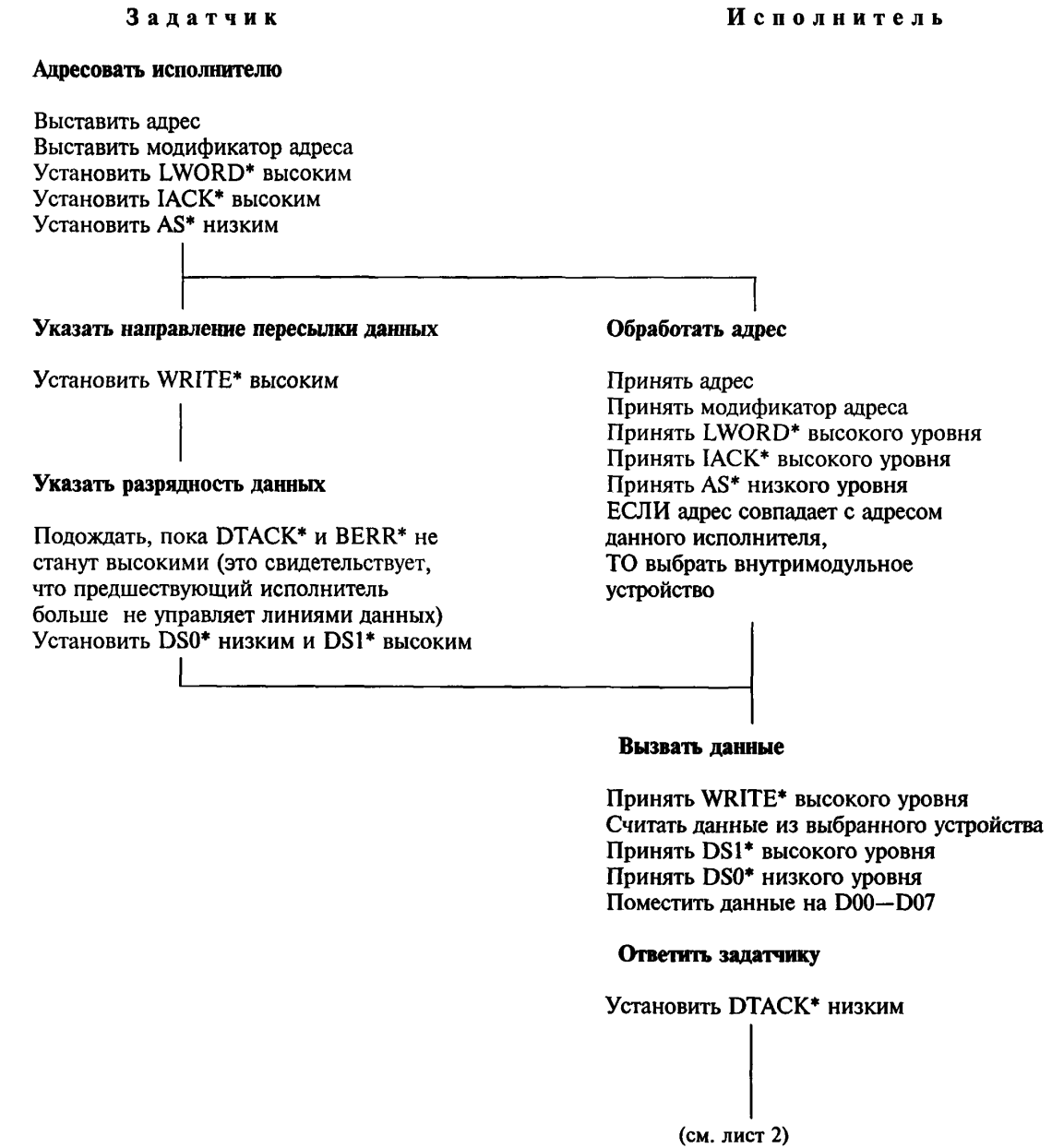
Рисунок 2.8, лист 1 — Пример однобайтового цикла считывания
