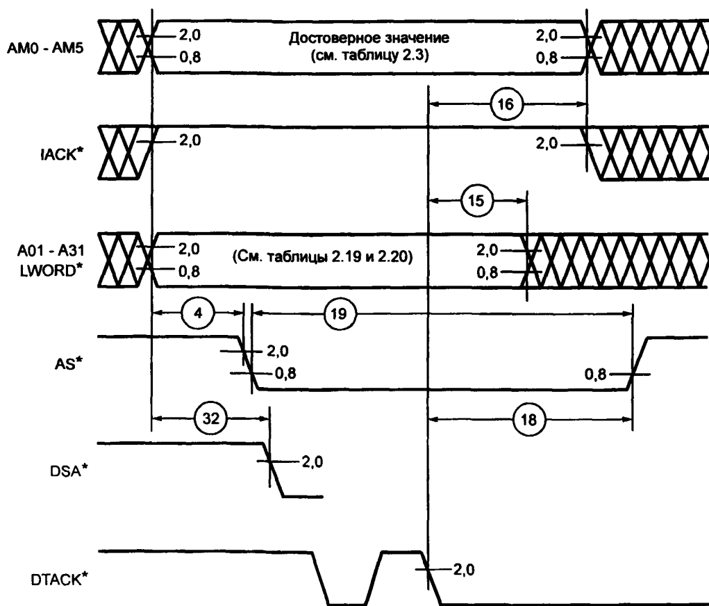
Значения напряжения пороговых уровней указаны в вольтах
