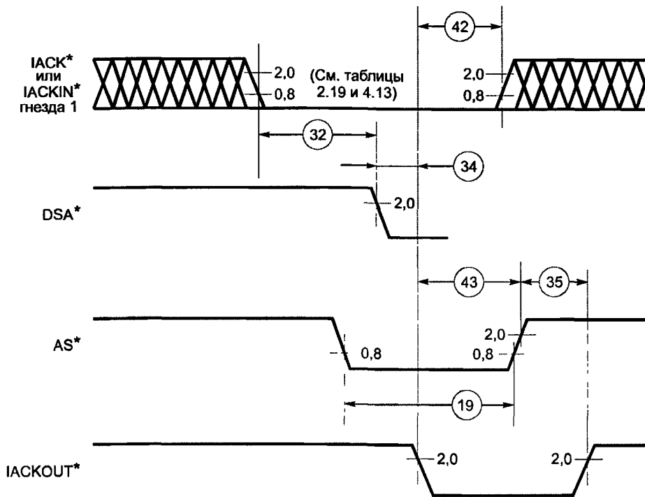
Значения напряжения пороговых уровней указаны в вольтах
