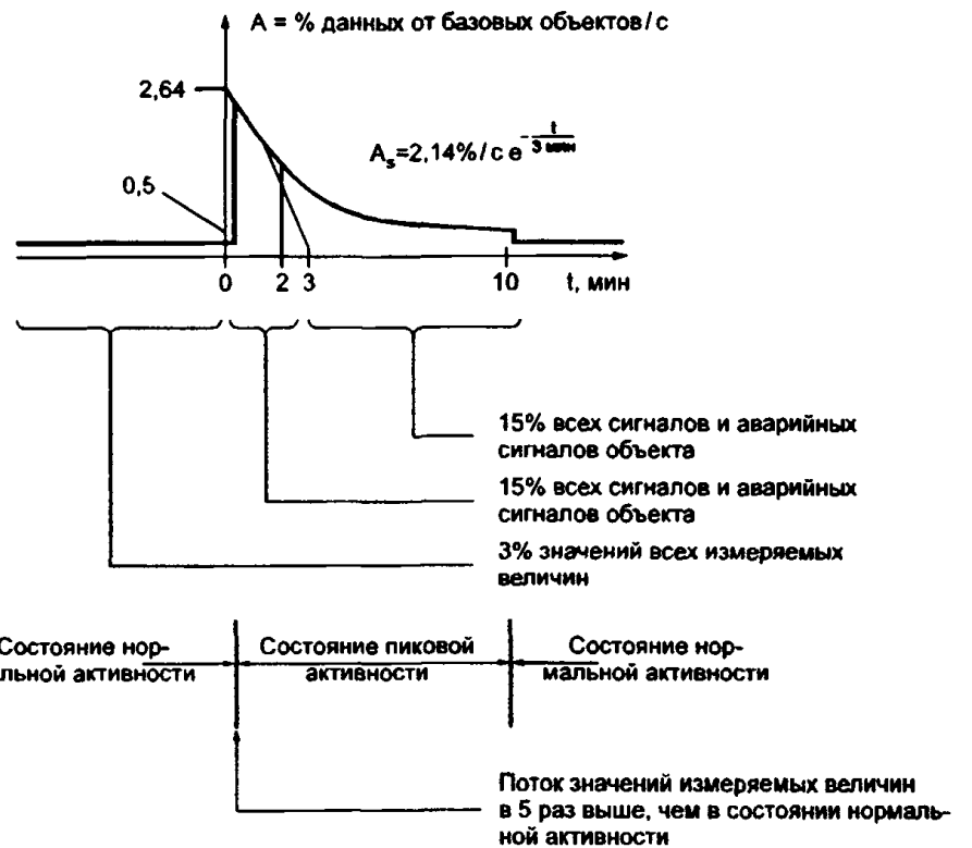
Рисунок А.1 — Определение расчетного потока данных
