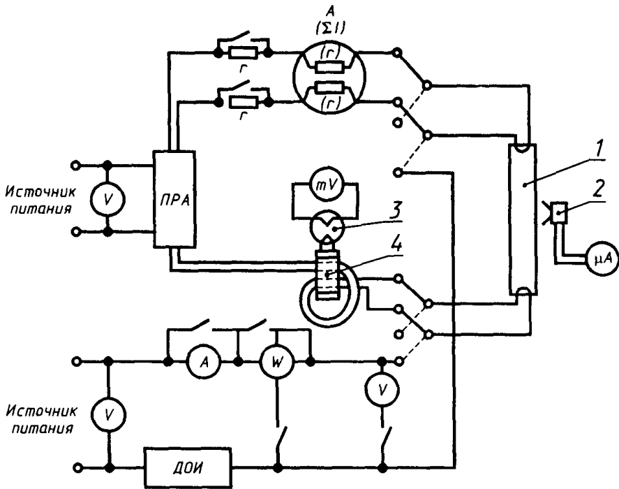
1 — номинальная лампа, 2 — фотозлемент, 3 — термопреобразователь, 4 — трансформатор тока
