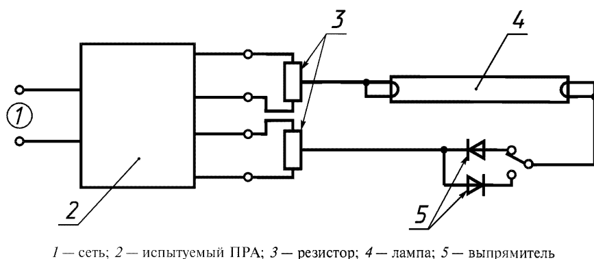
Рисунок 1 — Схема проверки выпрямляющего эффекта
