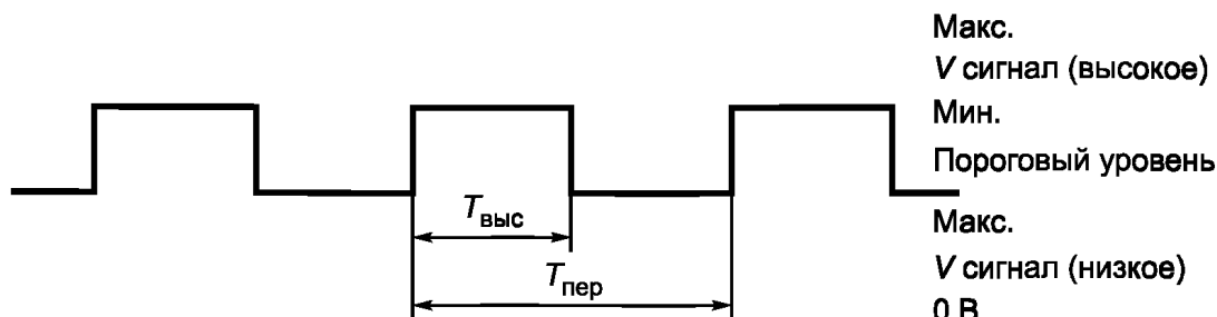
Типичный ШИМ сигнал
