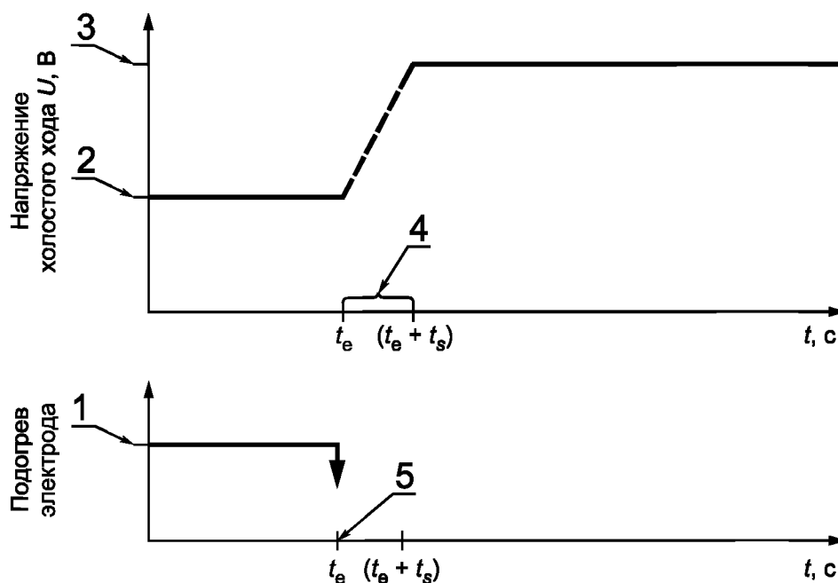
Рисунок 2.1 — ПРА, который прекращает ток предварительного подогрева при повышении напряжения холостого хода
