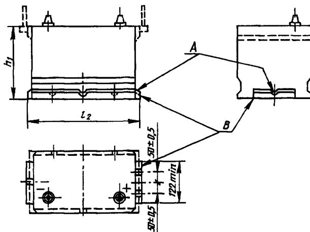
Дополнительные размеры батарей с допустимым поперемненным креплением, расположением выступов, выемок и выводов
