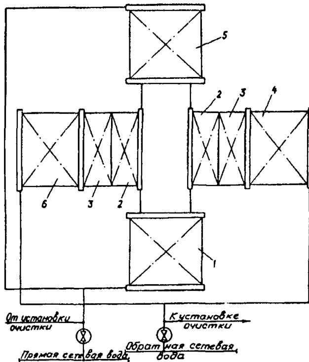
Рис. 3. Схема химической очистки котла ПТВМ-50:
