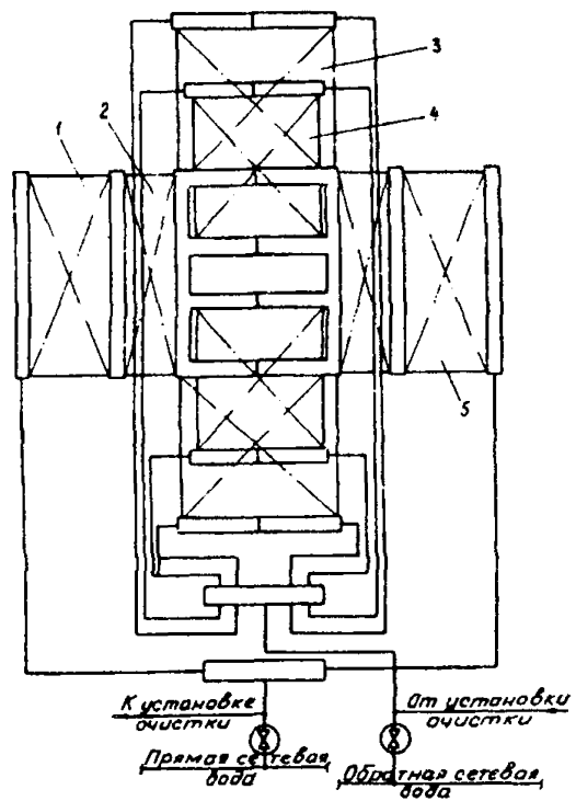
Рис. 6. Схема химической очистки котла ПТВМ-180 (двухходовая схема): 1 — задний экран; 2 — конвективный пучок; 3 — боковой экран; 4 — двухсветный экран; 5 — фронтальный экран; ⊗ — арматура закрыта
