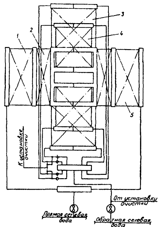
Рис. 7. Схема химической очистки котла ПТВМ-180 (четырёхходовая схема): 1 — задний экран; 2 — конвективный пучок; 3 — боковой экран; 4 — двухсветный экран; 5 — фронтальный экран; ⊗ — арматура закрыта; —|— — заглушка
