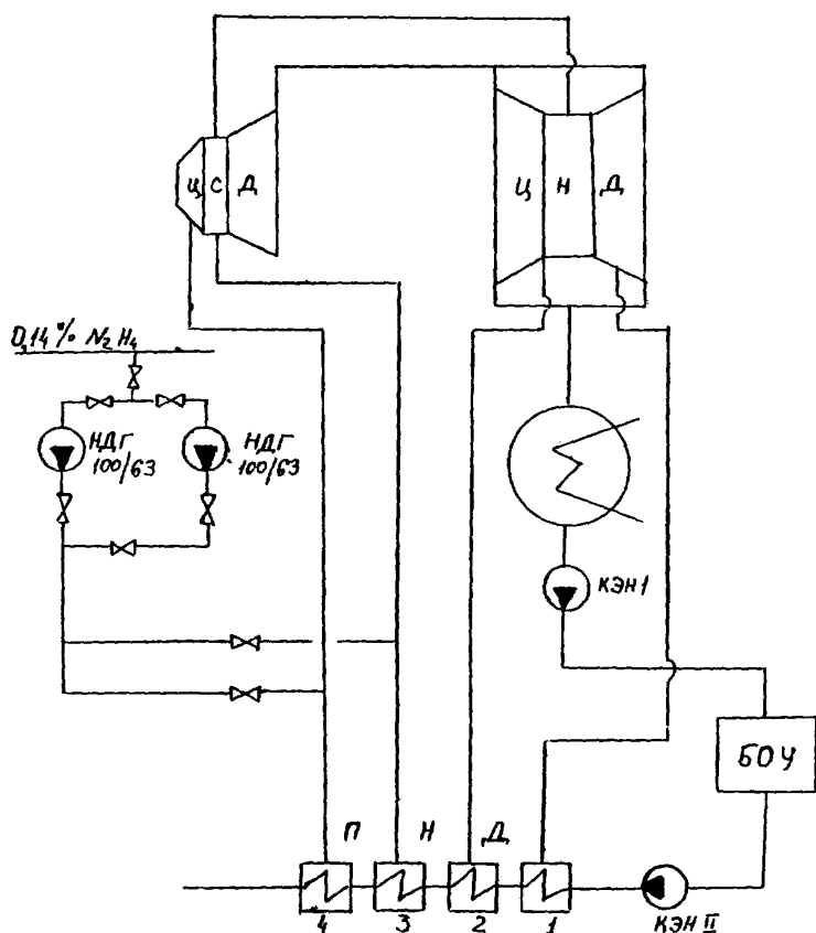
Рисунок 7 - Схема ввода гидрафина в паровое пространство ПНД энергоблока 300 МВт
