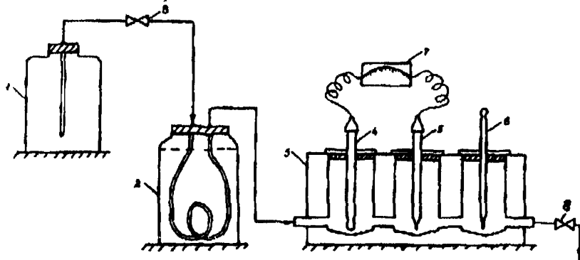
Установка для определения содержания натрия потенциометрическим методом:
