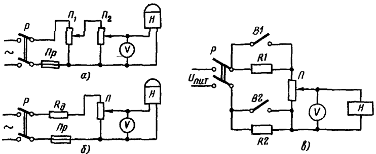
Рис. 17. Схемы для настройки реле ЭН и РН с малыми пределами уставок: а - с двумя потенциометрами П1 и П2; б - с потенциометром П и добавочным резистором R_з ; в - с автотрансформатором АТ и потенциометром П
