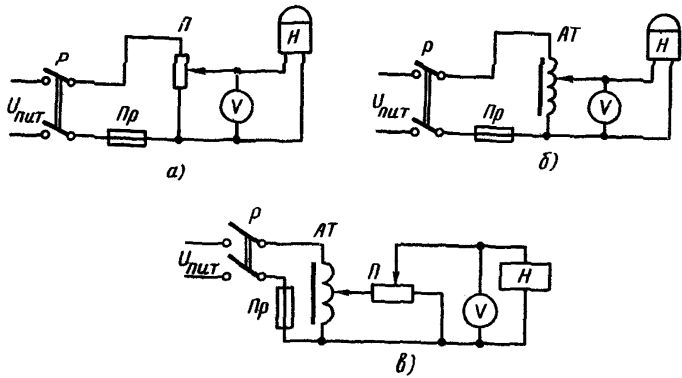
Рис. 16. Схемы регулирования напряжения: а - с потенциометром П; б - с автотрансформатором АТ; в - с двумя резисторами и потенциометром
