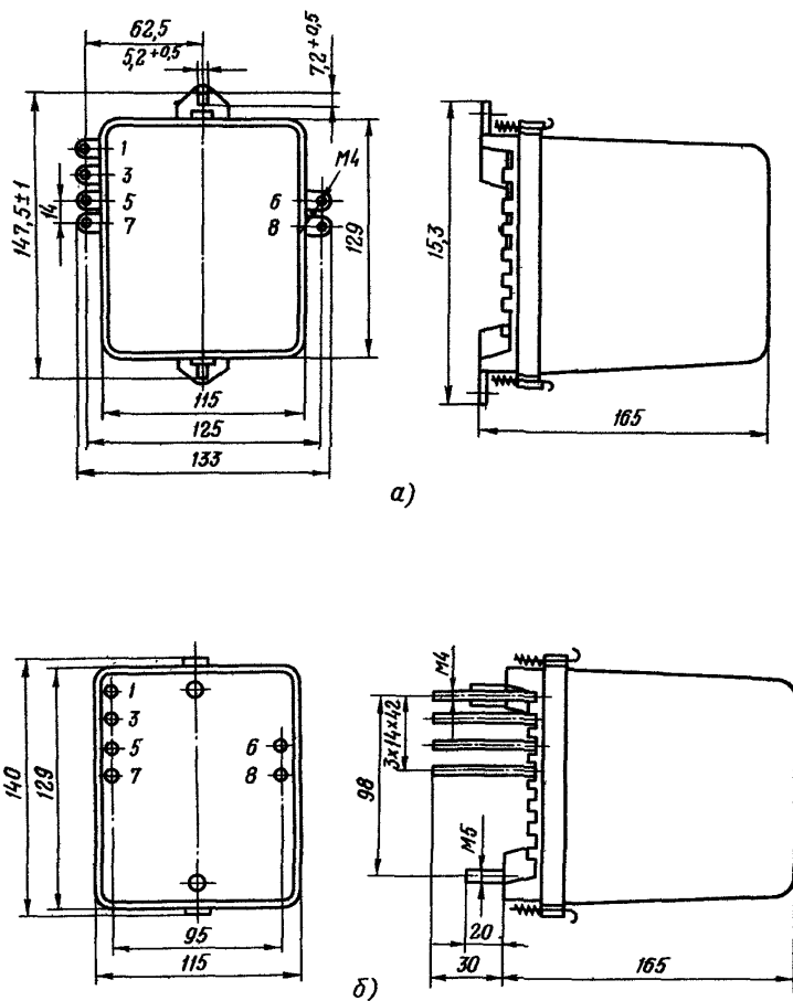
Рис.7. Габаритные и установочные размеры реле РНН-57, РН-58: а - переднее присоединение; б - заднее присоединение.
