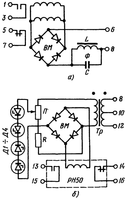
Рис.2. Схемы внутренних соединений: а - реле РНН-57; б - РН-58
