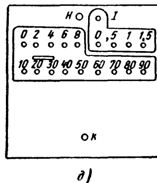
Рис. 3-3. Элементы реле сопротивления первой зоны защиты ДЗ-401 (ДЗ-501).
