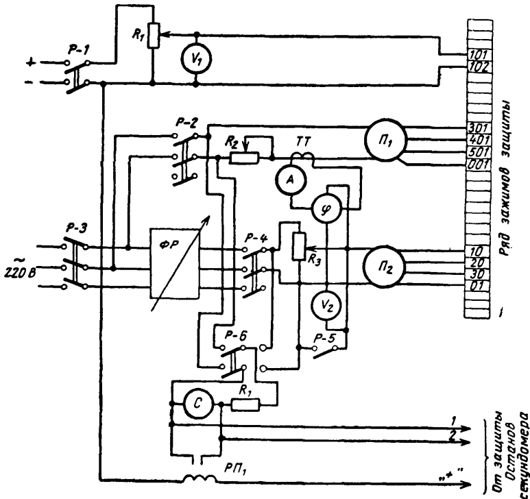
Рис. 4-6. Схема проверки защиты.
