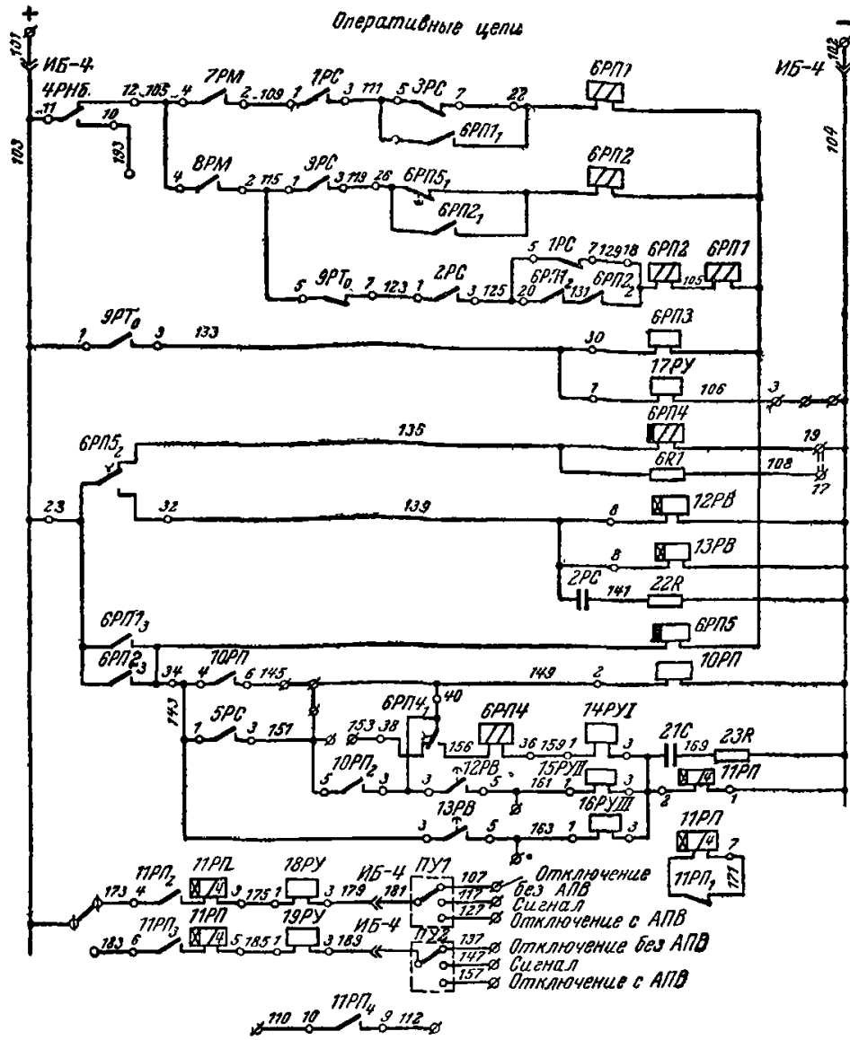
Рис. 1-1. Принципиальная схема защиты типа ПЗ-153 (положение
