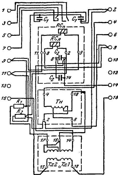
Монтажная схема
