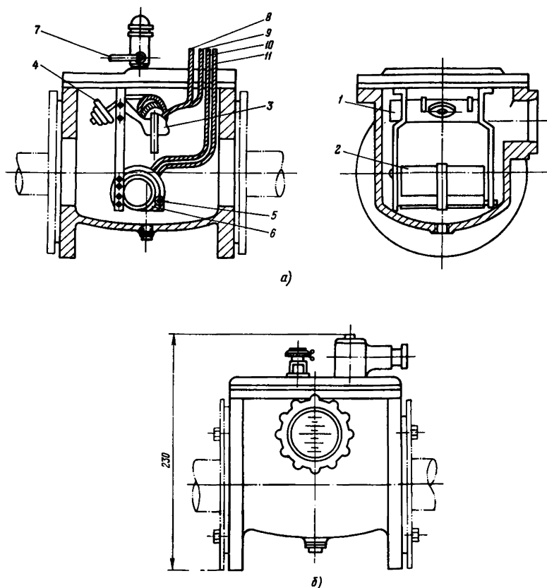
Рис.2. Газовое реле ПГЗ-22: а - конструкция; б - внешний вид
