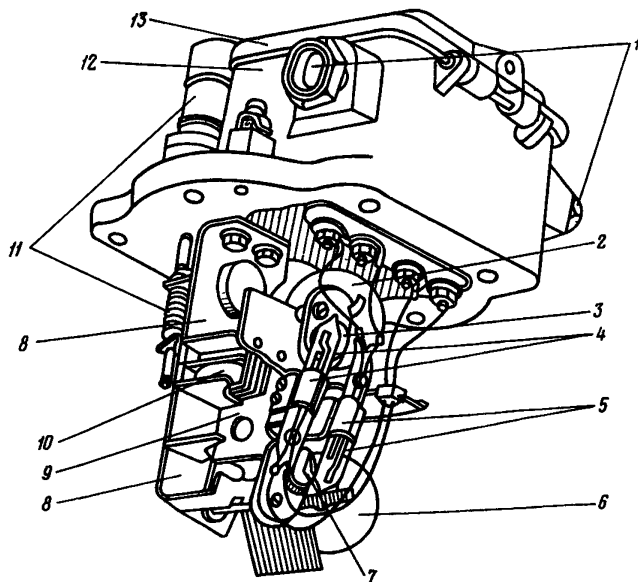
Рис.4. Объемная часть газового реле BF 80/Q (BF 50/I0)
