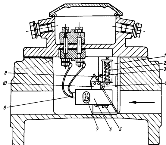
Рис.5. Струйное реле \ddot{U}FR\ 25/10
