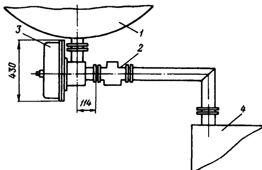
Рис.8. Схема размещения отсечного клапана на трансформаторе
