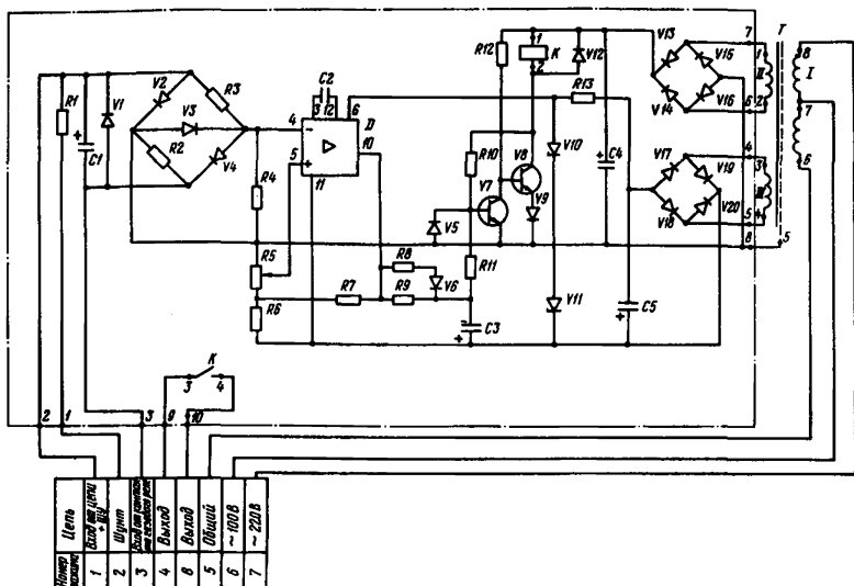
Рис.ПЗ.1. Принципиальная электрическая схема устройства КИЗ-1
