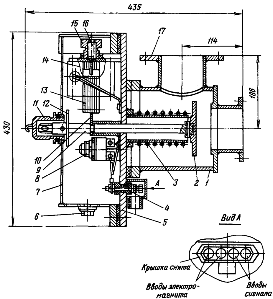
Рис.9. Конструкция отсечного клапана
