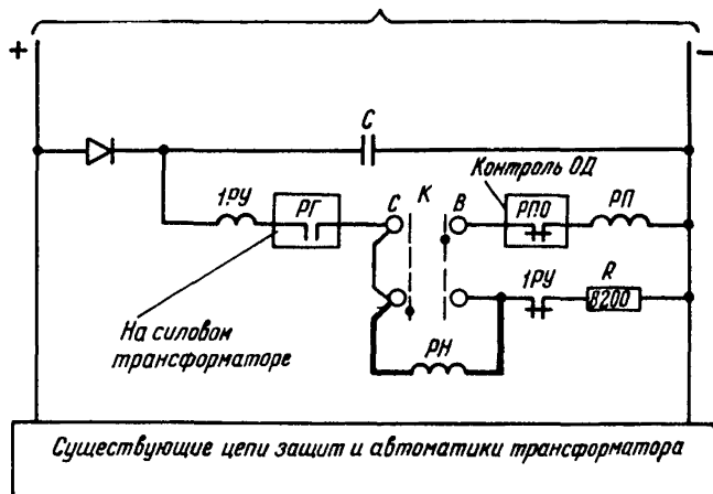
Рис.ПЗ.2. Схема для контроля понижения сопротивления изоляции на подстанциях с переменным оперативным током
