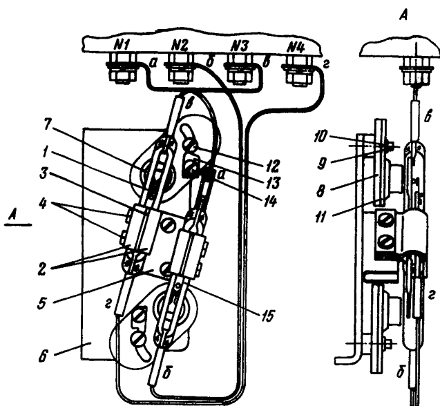
Рис.П4.1. Контактный узел реле BF 80/Q
