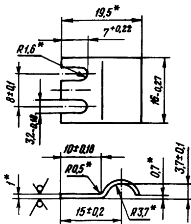
Рис.П4.3. Конструкция фиксирующих скоб
