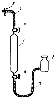
Рис.10. Прибор для отбора проб газа
