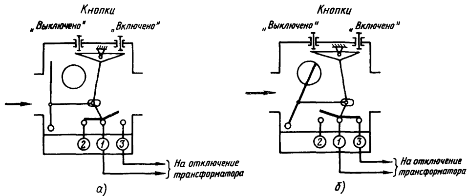
Рис.7. Функциональная схема реле RS - 1000: а - в нормальном режиме; б - в режиме срабатывания
