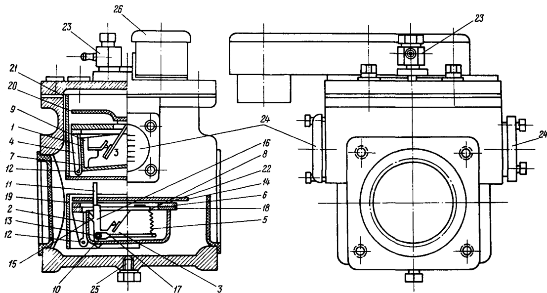
Рис.3. Газовое реле РГЧЗ-66:
