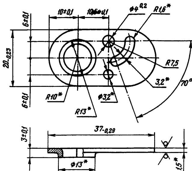
Рис.П4.2. Конструкция держателя
