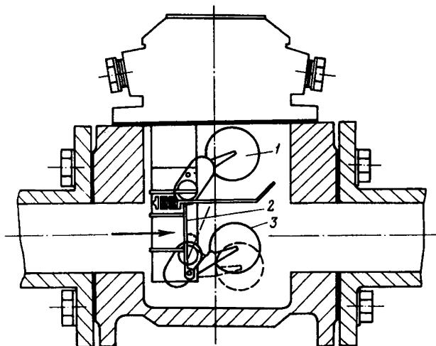
Рис.І. Газовое реле
