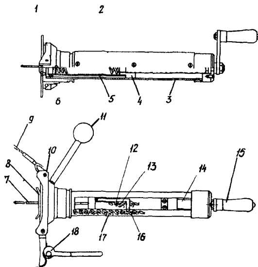
Рис.1. Общий вид прибора для определения степени загибания древесины опор:
