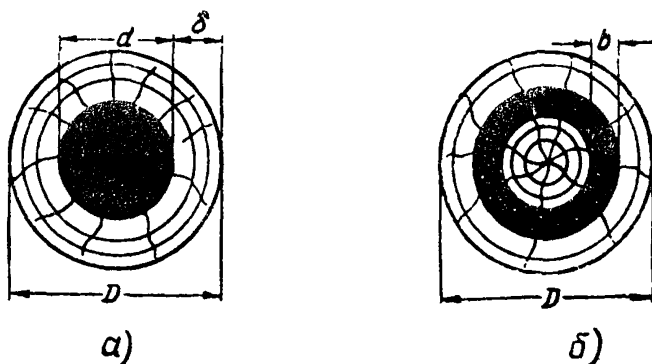
Рис.1. Условное сечение детали деревянной опоры: а - при полном внутреннем загнивании; б - при не- полном внутреннем загнивании
