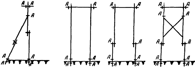
Рис.2. Опасные сечения деревянных опор: А - место опасного сечения
