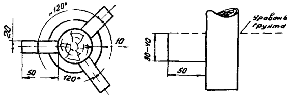
Рис.3. Размеры (см) и расположение ямок, выкапываемых вокруг пазышка при определении степени загнивания древесины опоры ниже уровня земли
