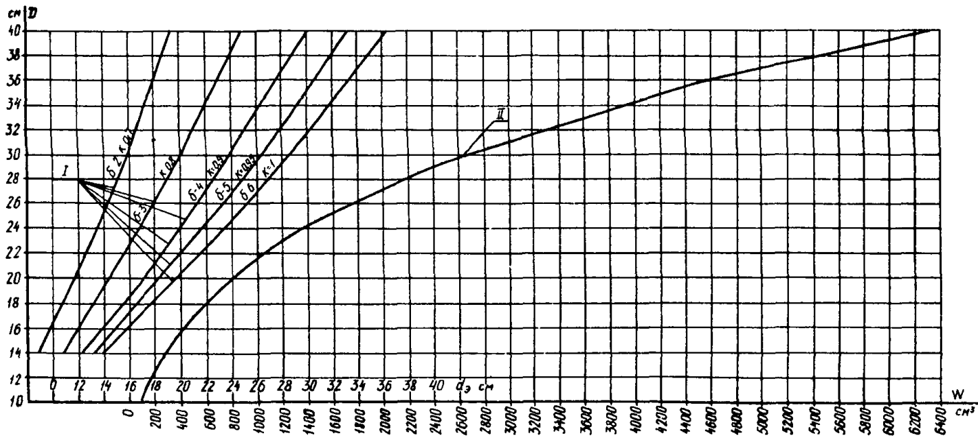
Рис.2. Кривые зависимости эквивалентных диаметров и моментов сопротивлений
