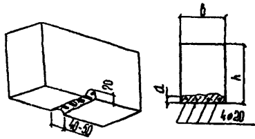
Рис. 3. Продольная арматура в середине пролета
