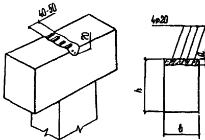
Рис. 4. Продольная арматура над опорой
