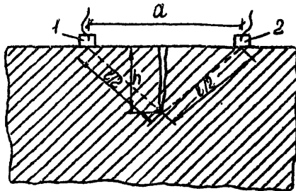
Рис. 1. Определение глубины трещины в конструкции: 1 — излучатель; 2 — приемник
