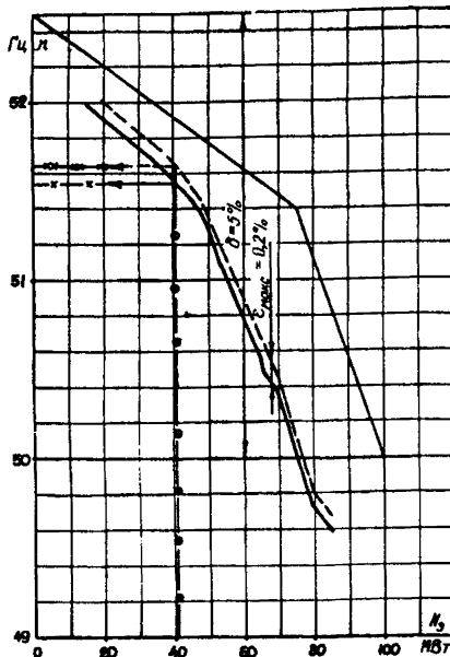
Рис.15. Суммарная статистическая характеристика турбины (на примере турбины № 8 Минской ТЭЦ-3)
