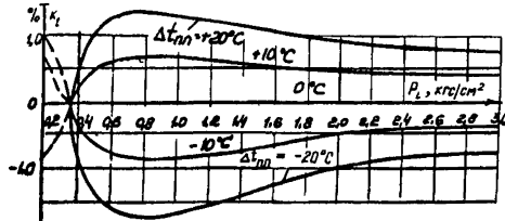
Рис. 18. Дополнительный поправочный коэффициент к давлениям пара в отборах от температуры в линии горячего промпарегрева:
