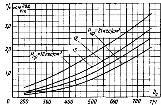
г) На отклонение подогревателей высокого давления
