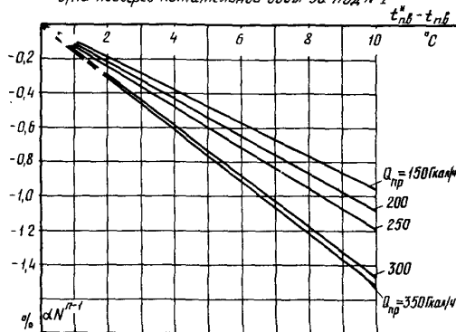
в) На недогрев питательной воды за ПВД №1
