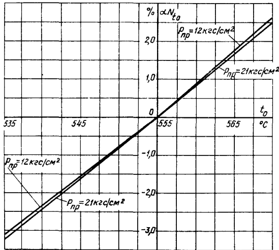
в) На отклонение температуры свежего пара от номинальной
