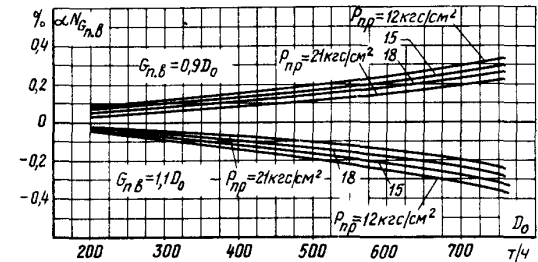
б) На отклонение расхода питательной воды от номинального
