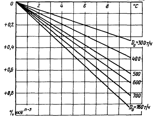
ж) На недогрев питательной воды за ПВД №3
