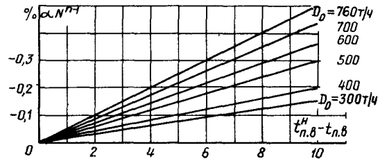
е) На недогрев питательной воды за ПВД №2
