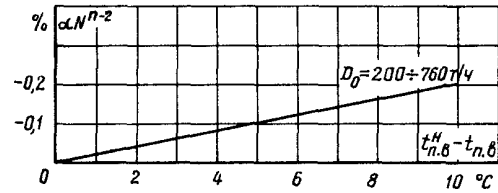
е) На недогрев питательной воды за ПВД №2
