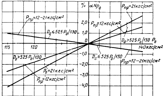
а) На отклонение давления свежего пара от номинального
