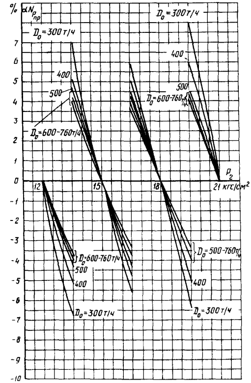
з) На отклонение давления отработанного пара от номинального
