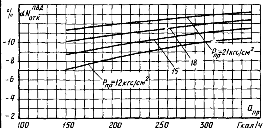
б) На отключение ПВД
