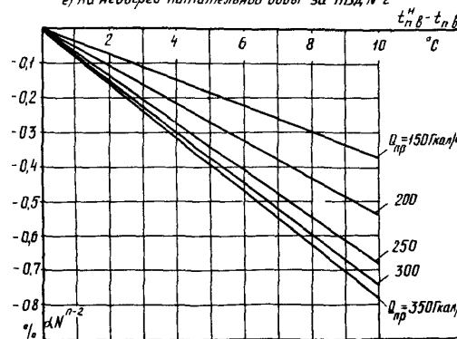
е) На недогрев питательной воды за ПВД №2
