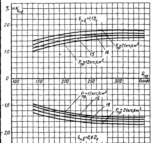
г) На отклонение расхода питательной воды
