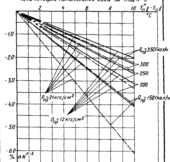
ж) На недогрев питательной воды за ПВД №3
