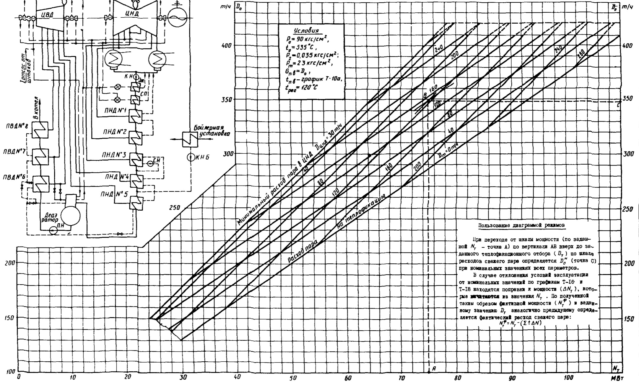
Принципиальная тепловая схема
