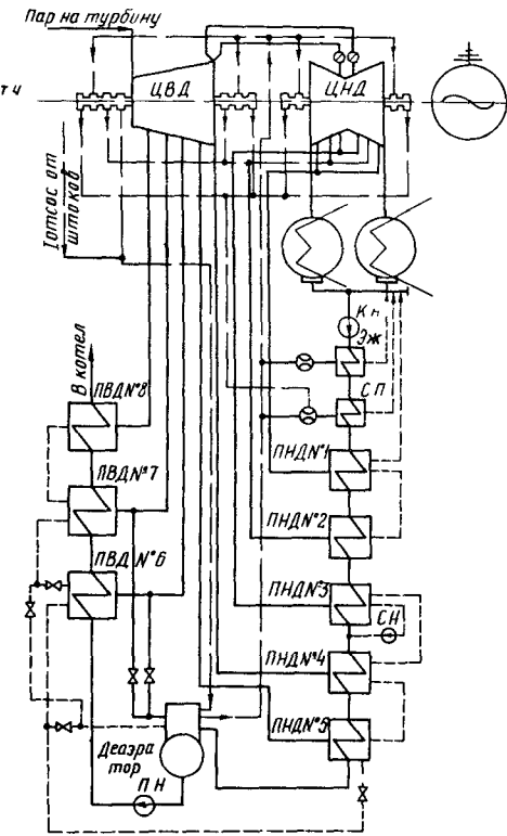
Принципиальная тепловая схема
