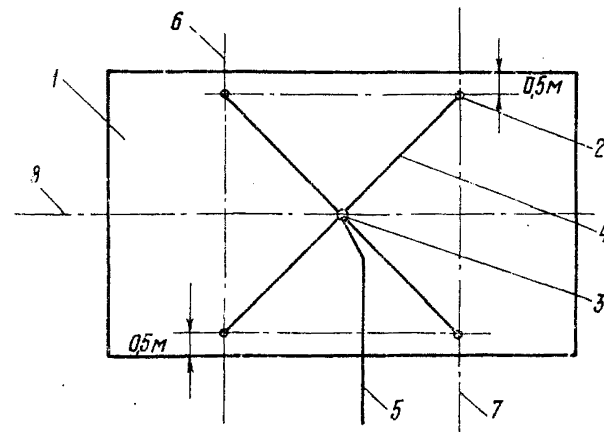
Схема расположения зондов для измерения давления пара в горловине конденсатора:
