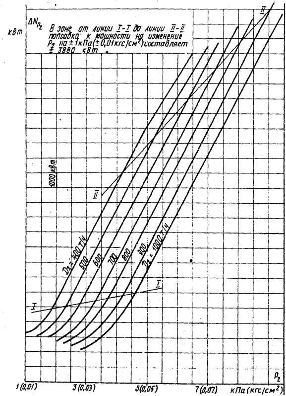
Рис. 10 ТИПОВАЯ ЭНЕРГЕТИЧЕСКАЯ ХАРАКТЕРИСТИКА КОНДЕНСАТОРА Поправка к мощности турбины К-500-240-2 ХТГЗ на отклонение давления отработанного пара Тип К-11520
