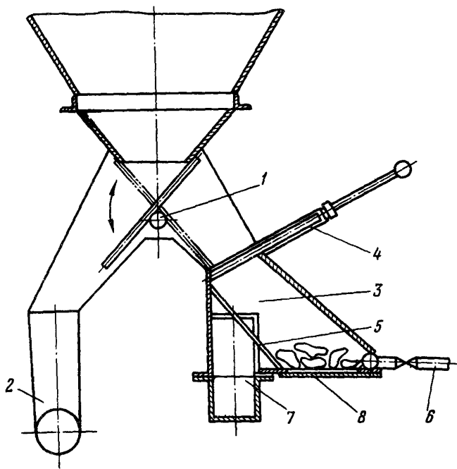
Рис.2.3. Узел эвакуации золы с конденсатоотводчиком и колосниковой решеткой:
