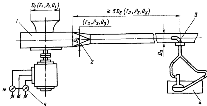
Рис.3.6. Схема установки для аэродинамических испытаний вентилятора:
