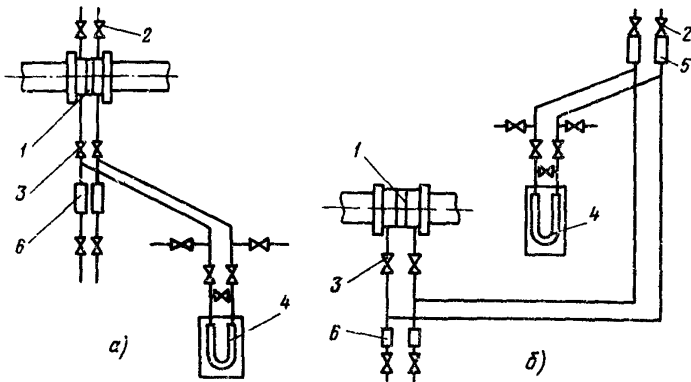
Рис.3.18 Схема соединительных линий для измерения расхода воды: а - установка дифманометра ниже диафрагмы; б - установка дифманометра выше диафрагмы; 1 - диафрагма; 2 - вентиль продувочный; 3 - вентиль; 4 - дифманометр; 5 - газосборник; 6 - отстойник
