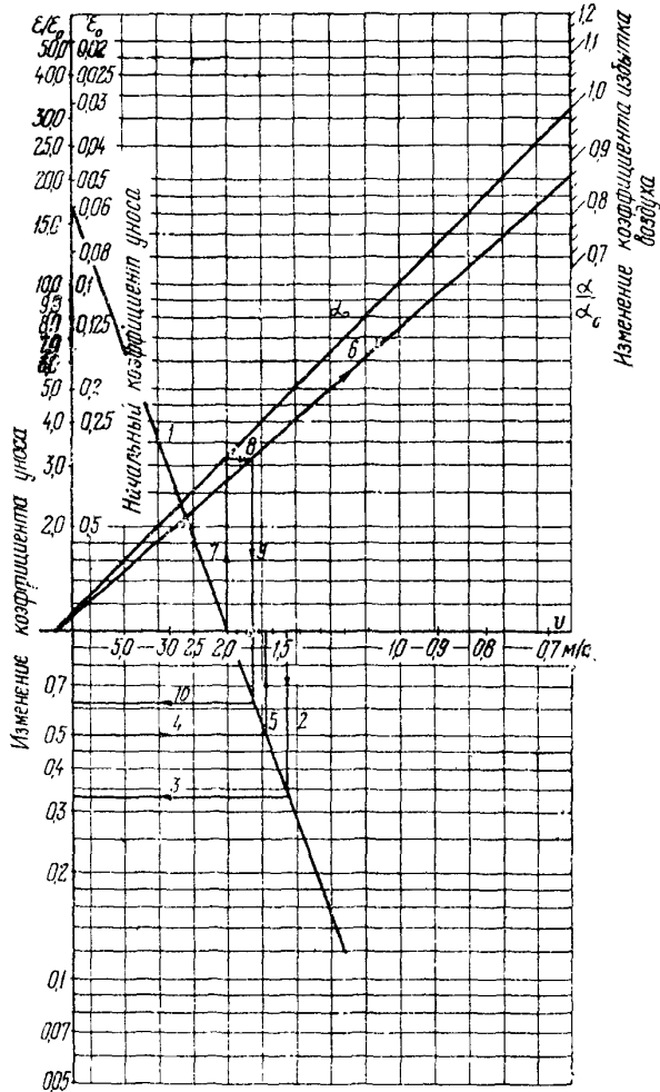
Рис.2. Расчет изменения степени очистки уходящих газов при изменении скорости газа (с учетом вторичного уноса для земли с УЭС < 5 \cdot 10^9 Ом·м)
