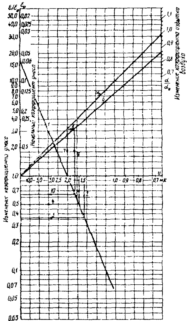
Рис. 1. Расчет изменения степени очистки уходящих газов при изменении скорости газа в электроfiltре (по формуле Дейча)
