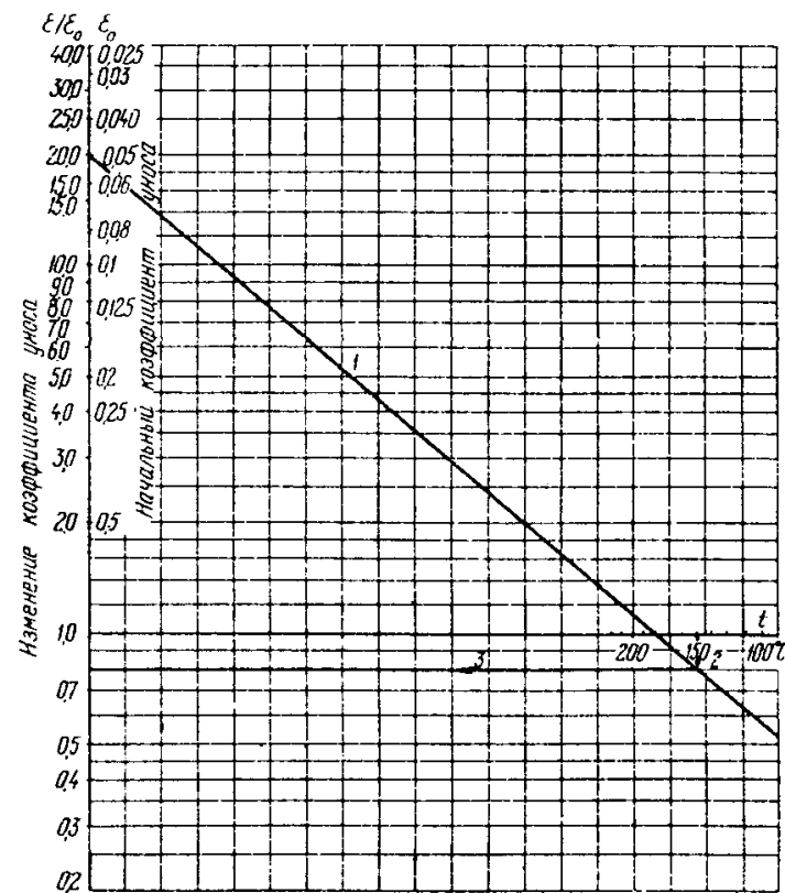
Рис. 6. Расчет изменения степени очистки уходящих газов при изменении температуры газов
