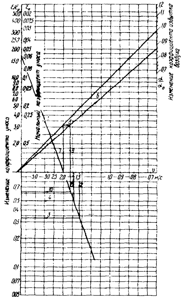
Рис. 2. Расчет изменения степени очистки уходящих газов при изменении скорости газа (с учетом вторичного уноса для золы с УЭС < 5 \cdot 10^9 \text{ Ом} \cdot \text{м} )
