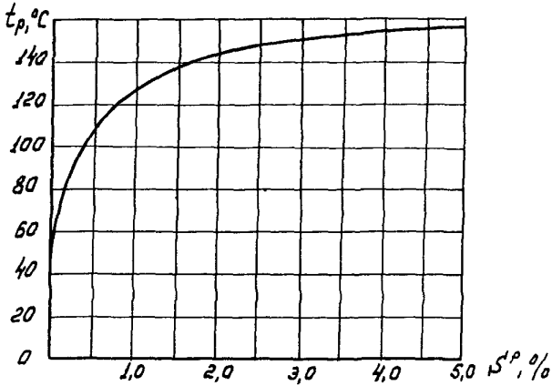
Рис. 1. Зависимость температуры точки росы дымовых газов от содержания серы в сжигаемом мазуте
