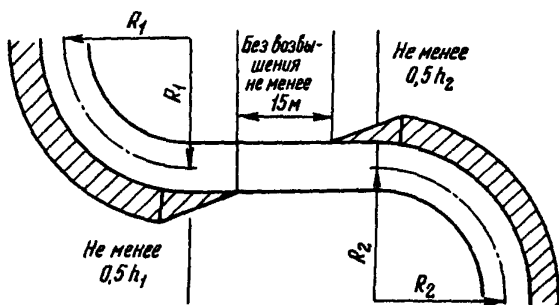
Рис.П.5. Устройство отводов возвышения при сопряжении обратных кривых и недостаточной длине прямой вставки между ними
