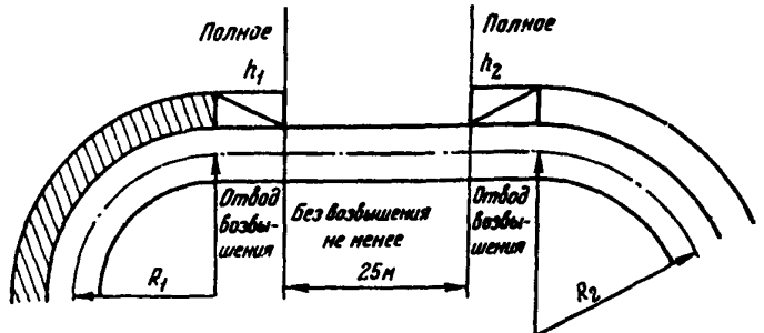
Рис.П.1.1. Устройство отводов возвышения при сопряжении кривых одинакового направления и достаточной длине прямой вставки между ними
