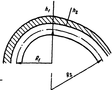
Рис.П.1.2. Устройство отводов возвышения при сопряжении кривых одинакового направления и недостаточной длине прямой вставки между ними
