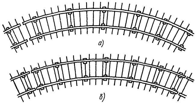
Рис.П.1.6. Металлические стяжки: а, б - соответственно по 5 и 7 стяжек на звено (рельсы длиной 12,5 м)
