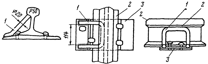
Рис.П.1.7. Металлические упорки: 1 - скоба (приваривается к подкладке строго по шаблону); 2 - рельс; 3 - подкладка
