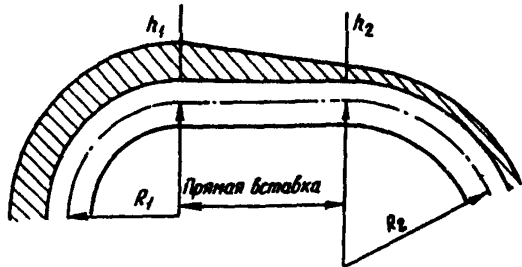
Рис.П.1.2. Устройство отводов возвышения при сопряжении кривых одинакового направления и недостаточной длине прямой вставки между ними
