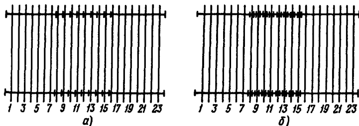
Рис. П.9. Схема расстановки пружинных противоугонов на рельсовых звеньях длиной 12,5 м:
