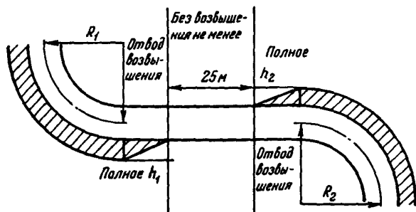
Рис.П.4. Устройство отводов возвышения при сопряжении обратных кривых и достаточной длине прямой вставки между ними
