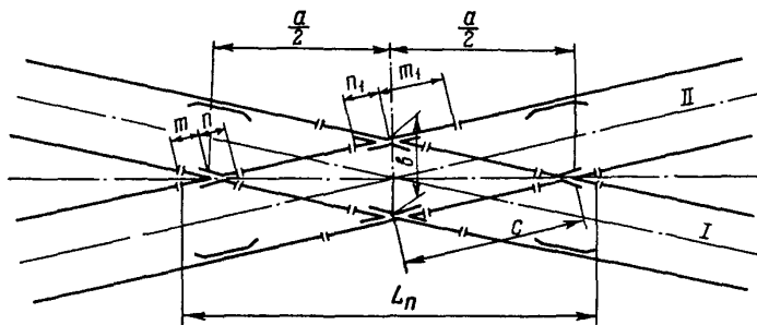
Рис. П. II. Схема глухого пересечения
