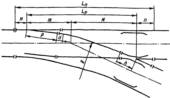
Рис. III.10. Схема обыкновенного стрелочного перевода
