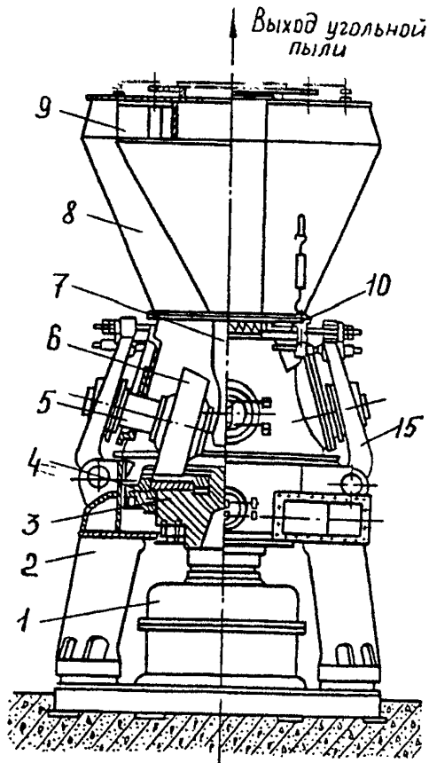
Рис. П1.1. Среднеходная мельница типа МВС с МВ: 1 — редуктор; 2 — корпус; 3 — стол; 4 — сопловой аппарат с подпорным кольцом; 5 — валок; 6 — бандаж; 7 — точка возврата грубой пыли; 8 — сепаратор; 9 — лопатки сепаратора; 10 — пружинный блок; 11 — электродвигатель; 12 — муфта; 13 — патрубок подвода сушильного агента; 14 — мигалка; 15 — рычаг; 16 — МВ; 17 — пылепровод
