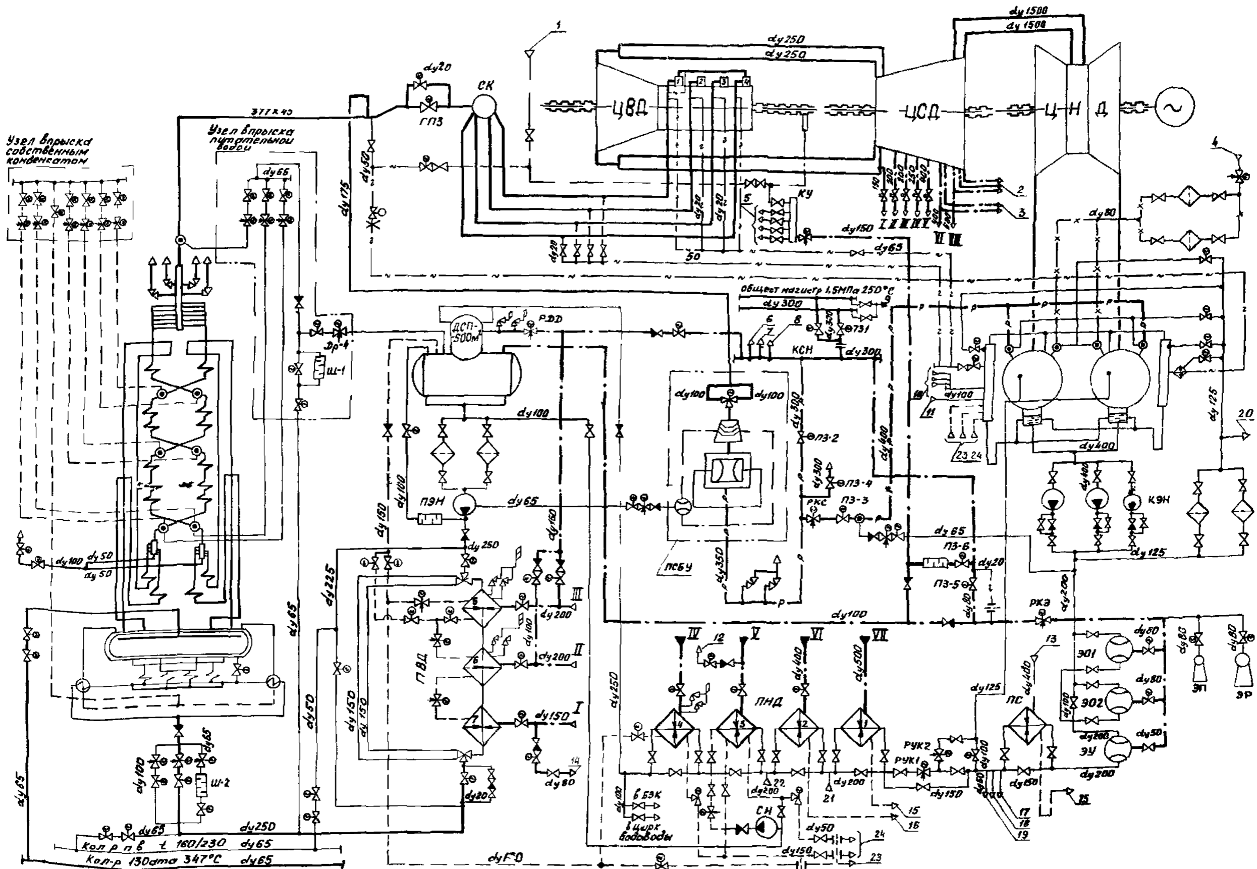
Рис.1. Типовая пусковая схема теплофикационного блока 110 МВт с газомасляным барабанным котлом и турбиной Т-110/120-130 ТМЗ:
