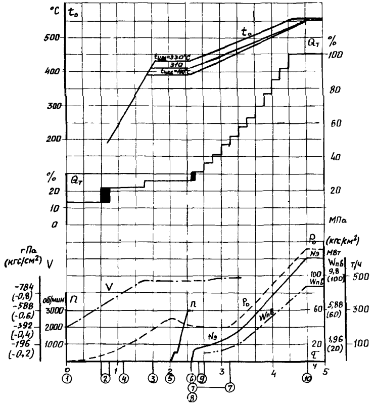
Рис. 4. График-задание пуска энергоблока из неустывшего состояния (температура металла верхя ЦВД в зоне регулирующей ступени 290-330 ^{\circ}\text{C} , продолжительность простоя 24-31 ч).
