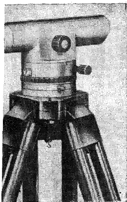
ис. 18. Нивелир Ni 050
