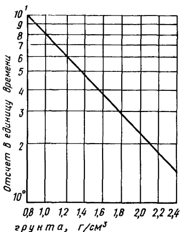
График градуировки радиоизотопного плотномера (тип. №)
